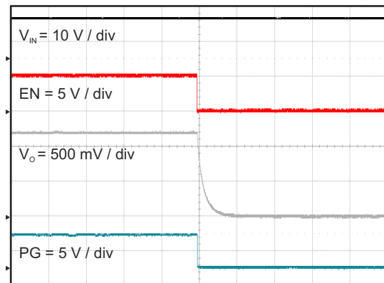
图 8-17. Shut Down Relative to EN Falling
