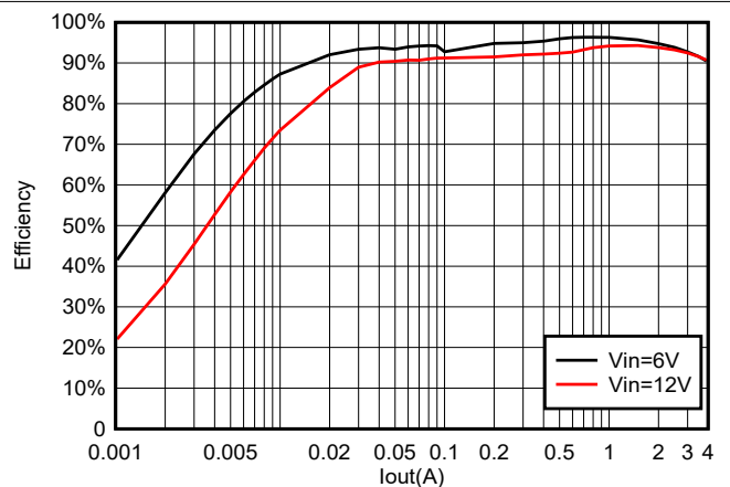
图 5-18. TPS564255B 在 3.3\text{V}_{\text{OUT}} 且使用 3.3\ \mu\text{H} 电感器时的效率
