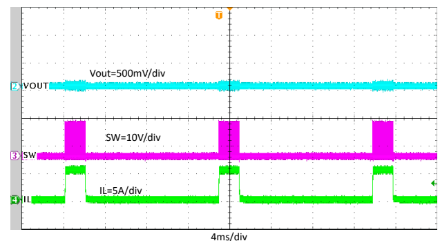
图 7-25. 输出硬短路断续
