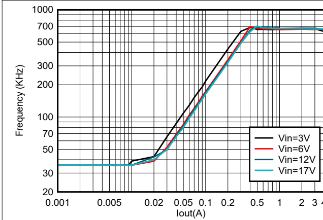
图 7-4. TPS564255B 频率与负载间的关系
