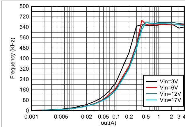
图 7-2. TPS564252B 频率与负载间的关系
