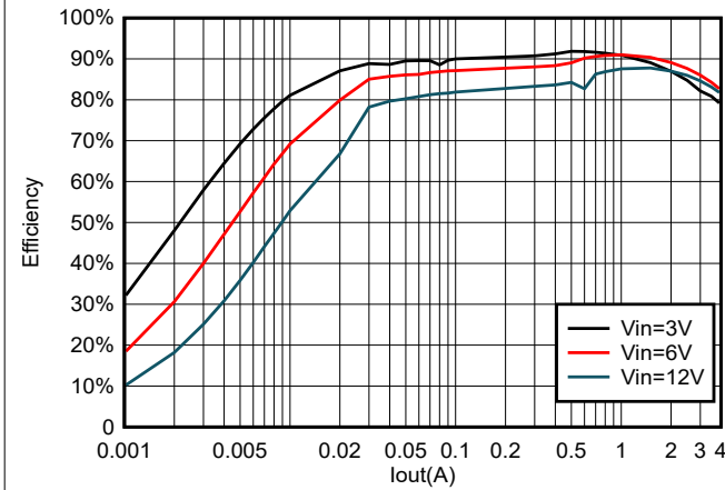
图 5-15. TPS564255B 在 1.05\text{V}_{\text{OUT}} 且使用 1.5\ \mu\text{H} 电感器时的效率
