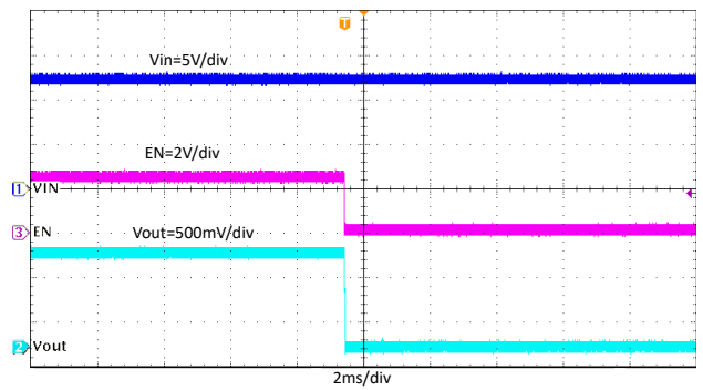
图 7-19. 通过 EN 关断, I_{OUT} = 4A
