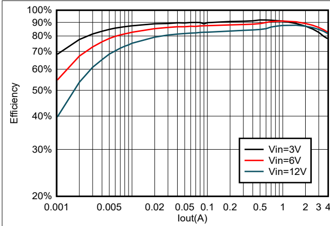
图 5-13. TPS564252B 在 1.05\text{V}_{\text{OUT}} 且使用 1.5\ \mu\text{H} 电感器时的效率
