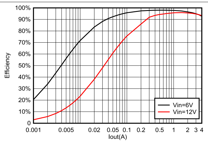
图 5-20. TPS564257B 在 5\text{V}_{\text{OUT}} 且使用 4.7\ \mu\text{H} 电感器时的效率
