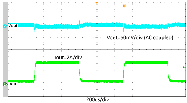
图 7-17. TPS564255B 瞬态响应, 0.4A 至 3.6A
