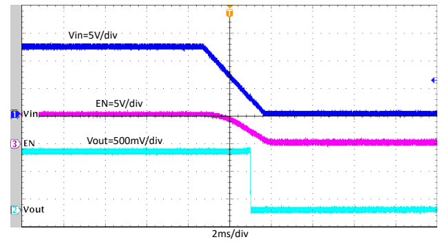
图 7-21. 在 V_{IN} 下降时关断, I_{OUT} = 4A
