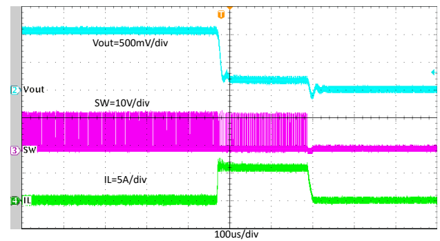
图 7-23. TPS564257B 正常运行至输出硬短路
