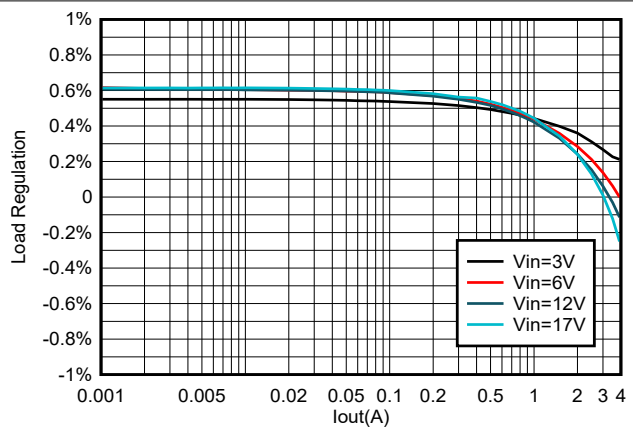
图 7-5. TPS564252B 负载调整率与负载间的关系
