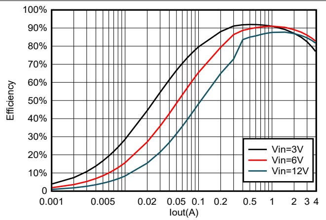
图 5-14. TPS564257B 在 1.05\text{V}_{\text{OUT}} 且使用 1.5\ \mu\text{H} 电感器时的效率
