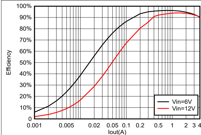
图 5-17. TPS564257B 在 3.3\text{V}_{\text{OUT}} 且使用 3.3\ \mu\text{H} 电感器时的效率
