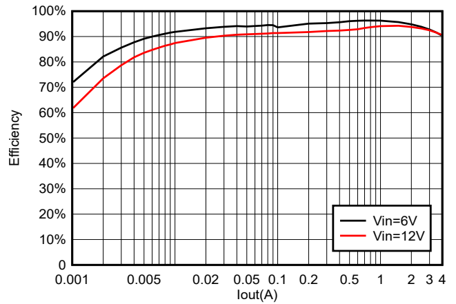
图 5-16. TPS564252B 在 3.3\text{V}_{\text{OUT}} 且使用 3.3\ \mu\text{H} 电感器时的效率
