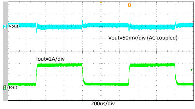
图 7-15. TPS564252B 瞬态响应, 0.4A 至 3.6A
