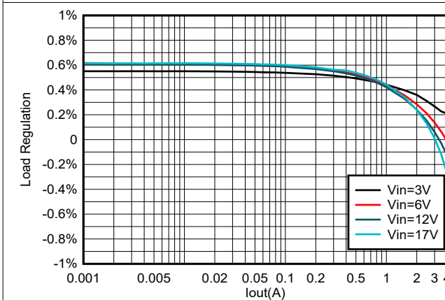
图 7-6. TPS564257B 负载调整率与负载间的关系
