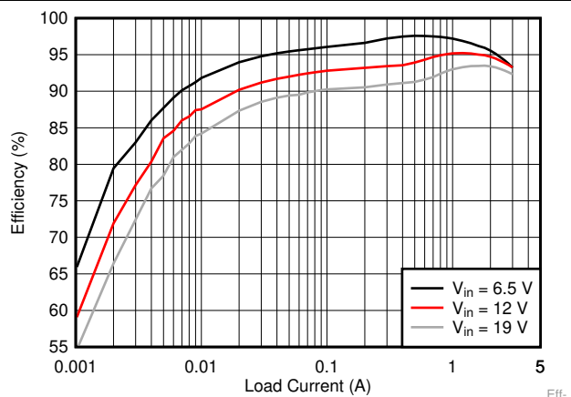
图 11. V_{OUT}=1.05\text{ V} Efficiency, L=1.5\text{ }\mu\text{H}
