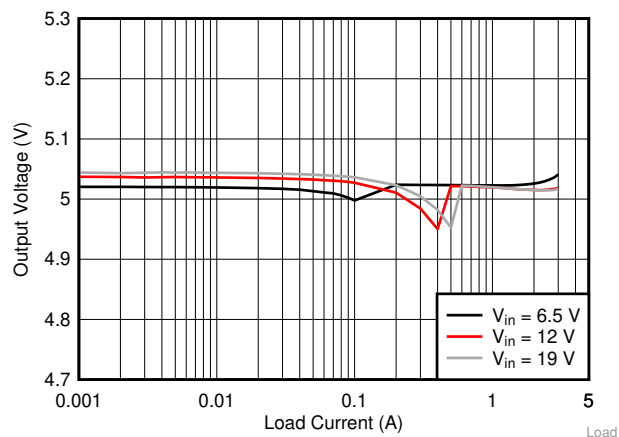
图 19. Load Regulation
