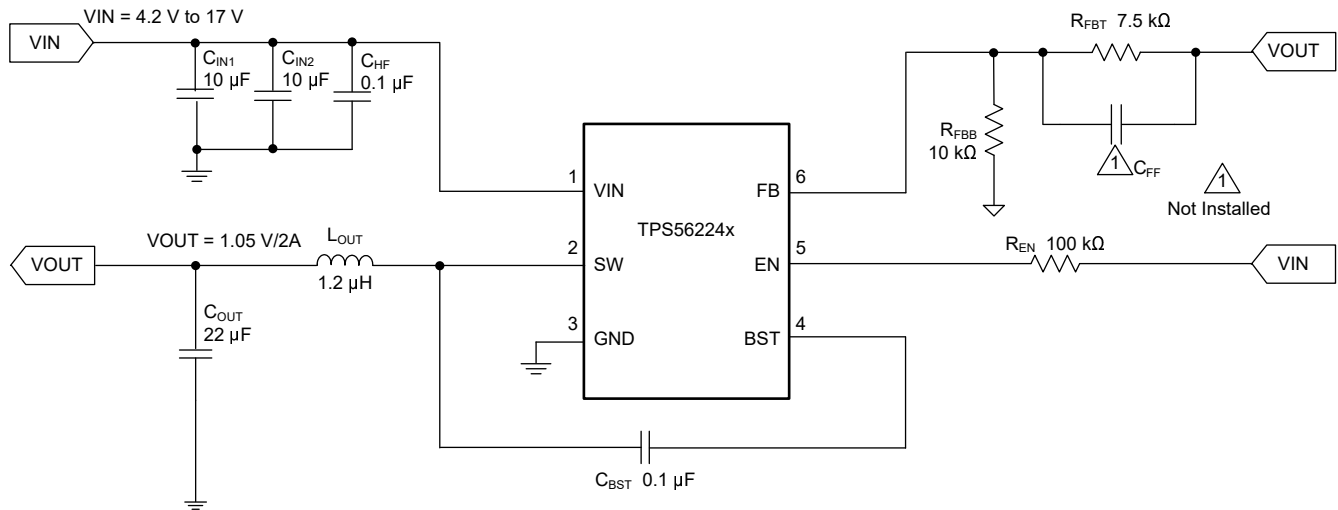
图 7-1. TPS56224xx 1.05V/2A 参考设计
