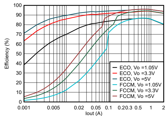
TPS56224xx 在 V_{in} = 12V 时的效率
