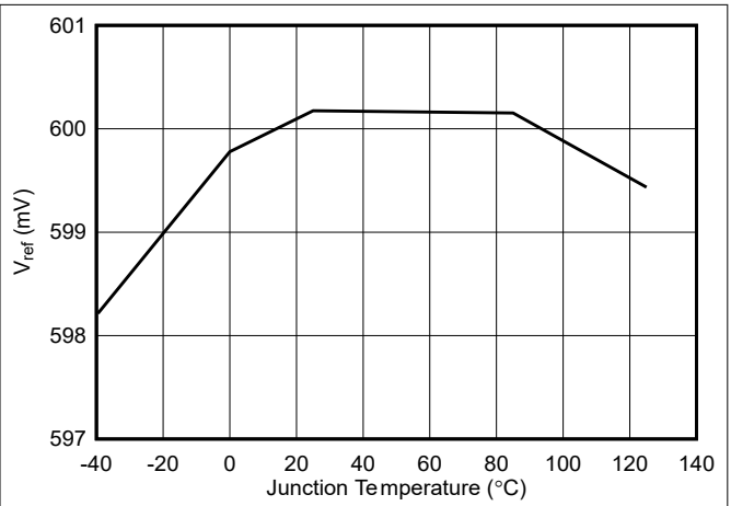
图 5-2. V_{ref} 电压
