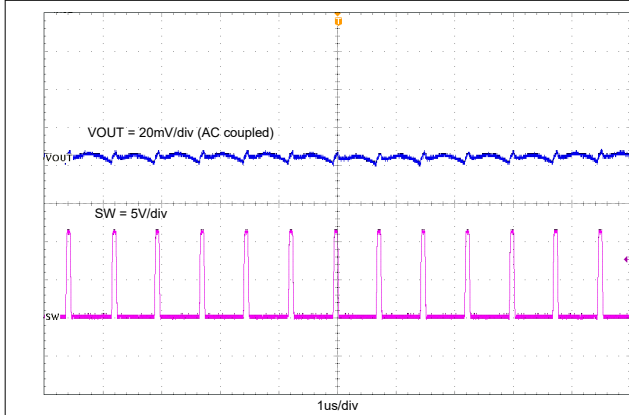
图 7-4. TPS562243 输出电压纹波 (2A 负载)
