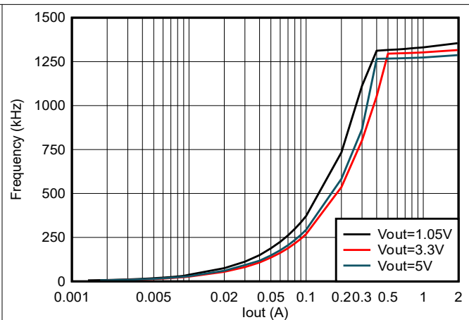
图 5-8. TPS562243 频率与负载间的关系
