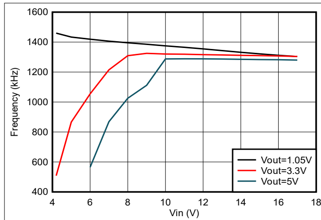
图 5-7. 2A 负载下频率与输入电压间的关系
