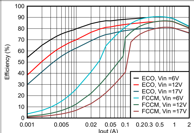
图 5-10. TPS56224x 在 1.05Vout 且使用 1.2uH 电感器时的效率
