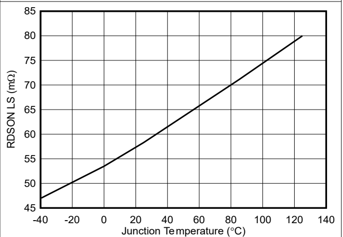
图 5-6. 高侧 R_{dson}
