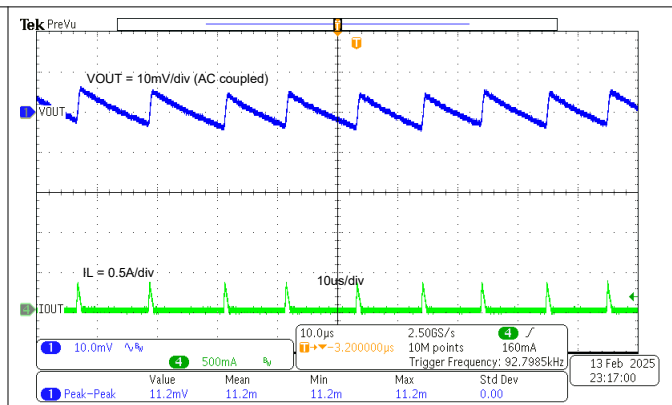
图 7-3. TPS561300EVM 输出电压纹波, I_{OUT} = 0.01A
