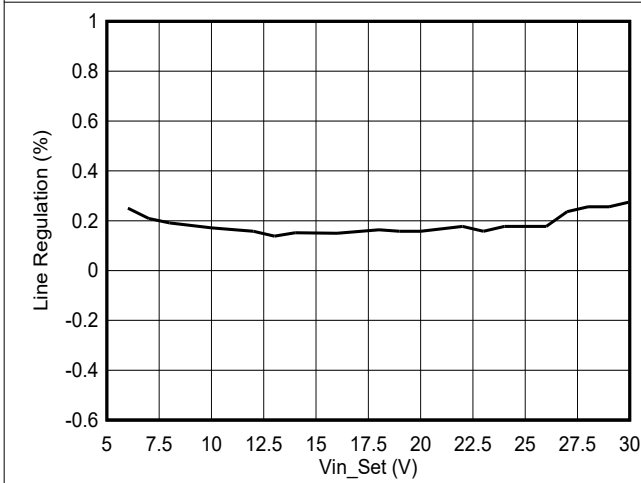
图 7-10. TPS561300EVM 线性调整率, I_{OUT} = 1A
