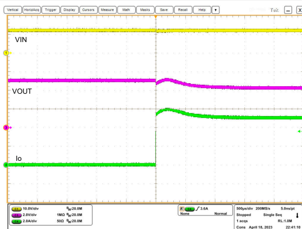
图 8-12. V_{IN} = 12V 、 V_{OUT} = 5V 、 R_{LOAD} = 0.8\Omega 、 R_{SNS} = 10m\Omega 时的输出电流波形，FPWM
