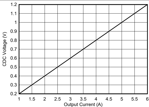
图 6-17. CDC 电压与输出电流间的关系, R_{SENSE} = 10m\Omega
