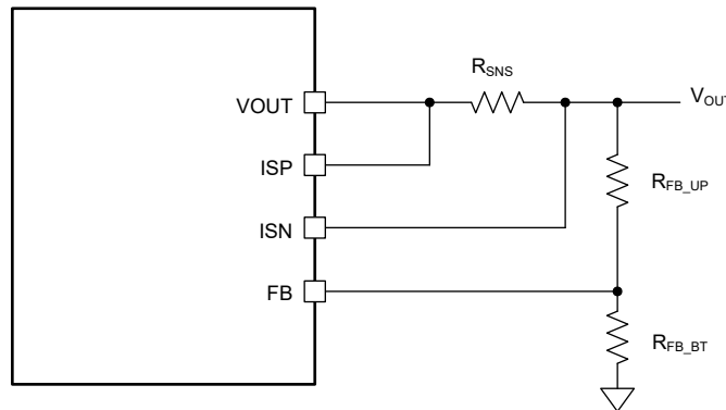
图 7-5. Output Voltage Setting
