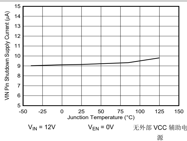
图 5-18. VIN 引脚关断静态电流与结温间的关系
