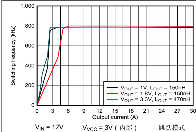
图 5-13. 800kHz 跳跃模式开关频率与输出电流间的关系
