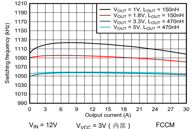
图 5-14. 1100kHz 开关频率与输出电流间的关系
