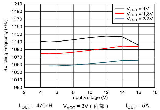
图 5-10. 1100kHz 开关频率与输入电压间的关系
