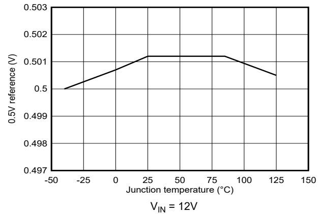
图 5-16. 0.5V 基准电压与结温间的关系
