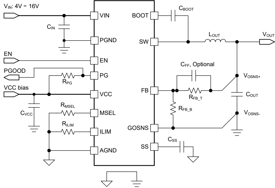
图 6-8. 具有外部 VCC 辅助电源的分离轨配置
