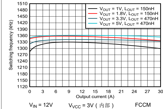
图 5-15. 1400kHz 开关频率与输出电流间的关系
