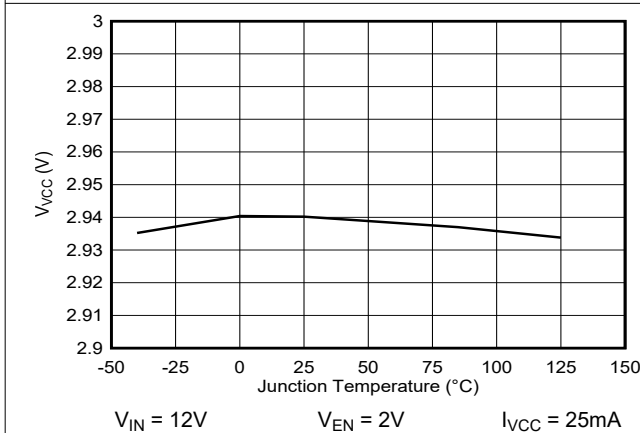
图 5-17. VCC 引脚输出电压与结温间的关系
