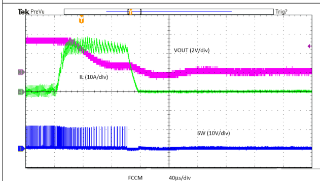
图 6-21. Overcurrent Protection
