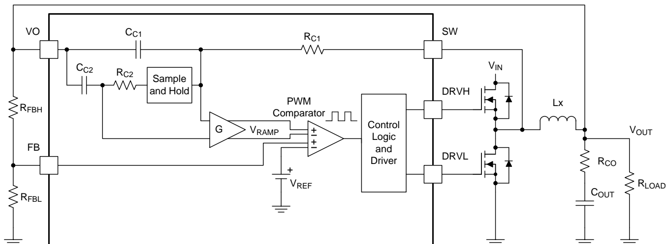
图 32. D-CAP3 Mode
