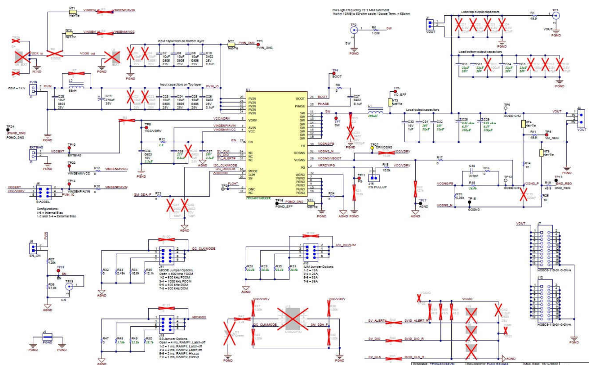
图 8-1. TPS548C26EVM 3.3-V 输出应用
