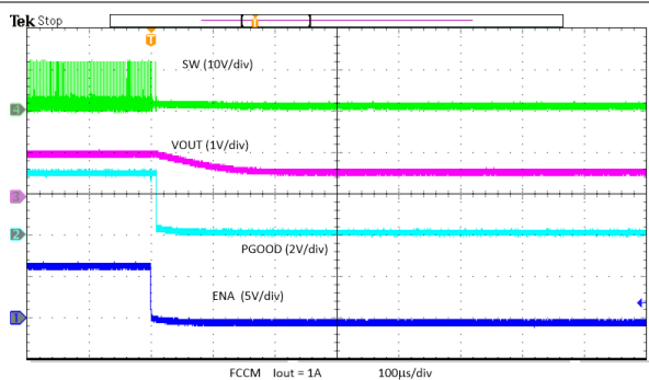
图 8-15. Prebias Power-Down
