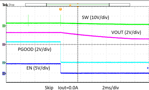
图 8-23. 使能预偏置断电，跳跃
