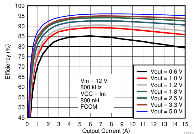
效率图
