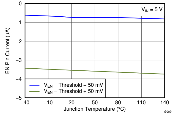
图 6-8. EN Pin Current vs Temperature
