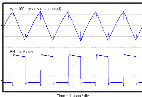
图 8-10. Input Ripple, IOUT = 7 A
