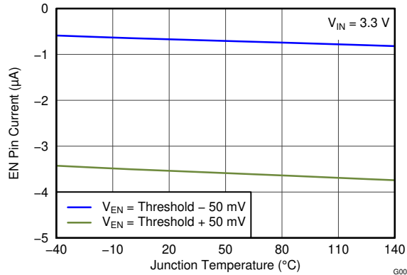
图 6-7. EN Pin Current vs Temperature
