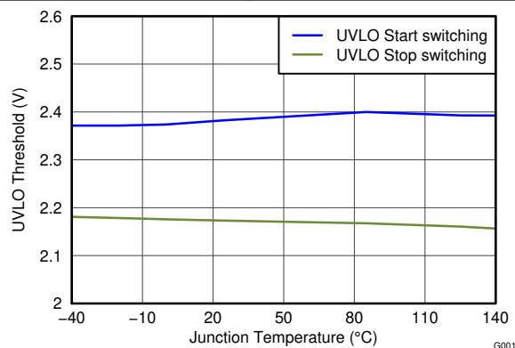
图 6-21. UVLO Threshold vs Temperature
