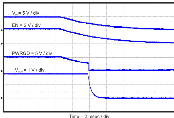
图 8-6. Power Down Relative To VIN
