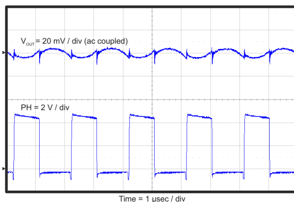
图 8-9. Output Ripple, IOUT = 7 A
