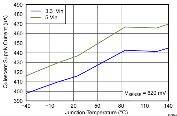
图 6-3. VIN Supply Current vs Temperature
