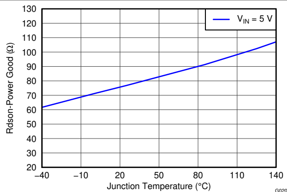
图 6-19. PWRGD Rdson vs Temperature
