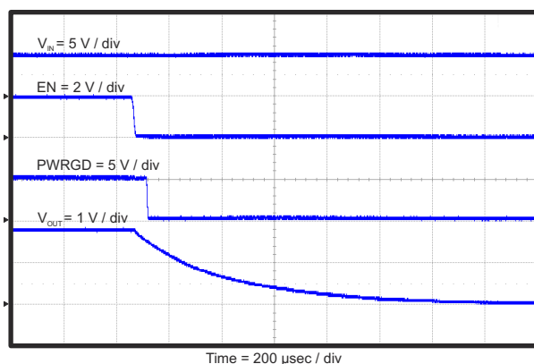
图 8-8. Power Down Relative To EN
