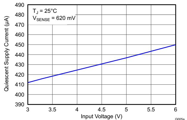
图 6-4. VIN Supply Current vs Voltage
