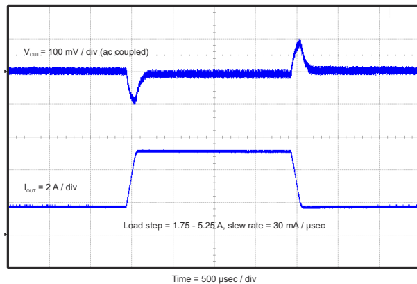
图 8-4. Transient Response, 3.5 A Step
