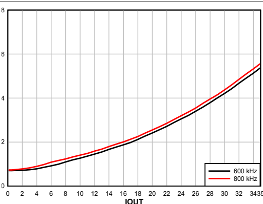
图 8-3. 功率耗散, FCCM, 内部 LDO
