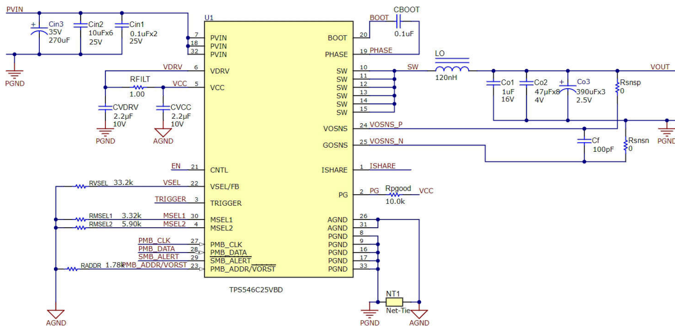
图 8-1. 1.2V、35A 输出应用
