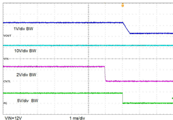
图 8-14. 控制关闭时的关断, 0A 负载
