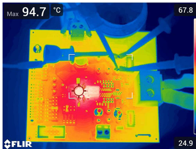
图 8-19. 热感图像，800kHz FCCM，35A 负载
