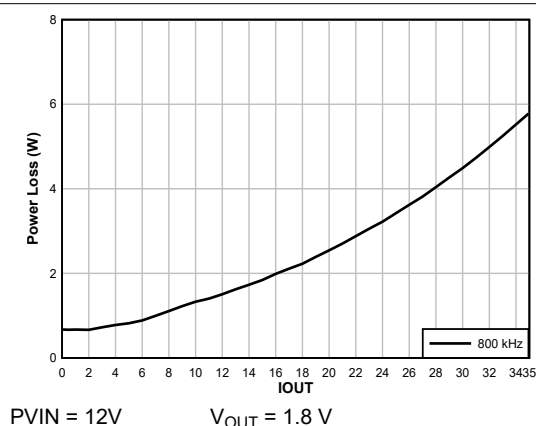
图 8-11. 功率耗散, FCCM, 外部 5V 辅助电源
