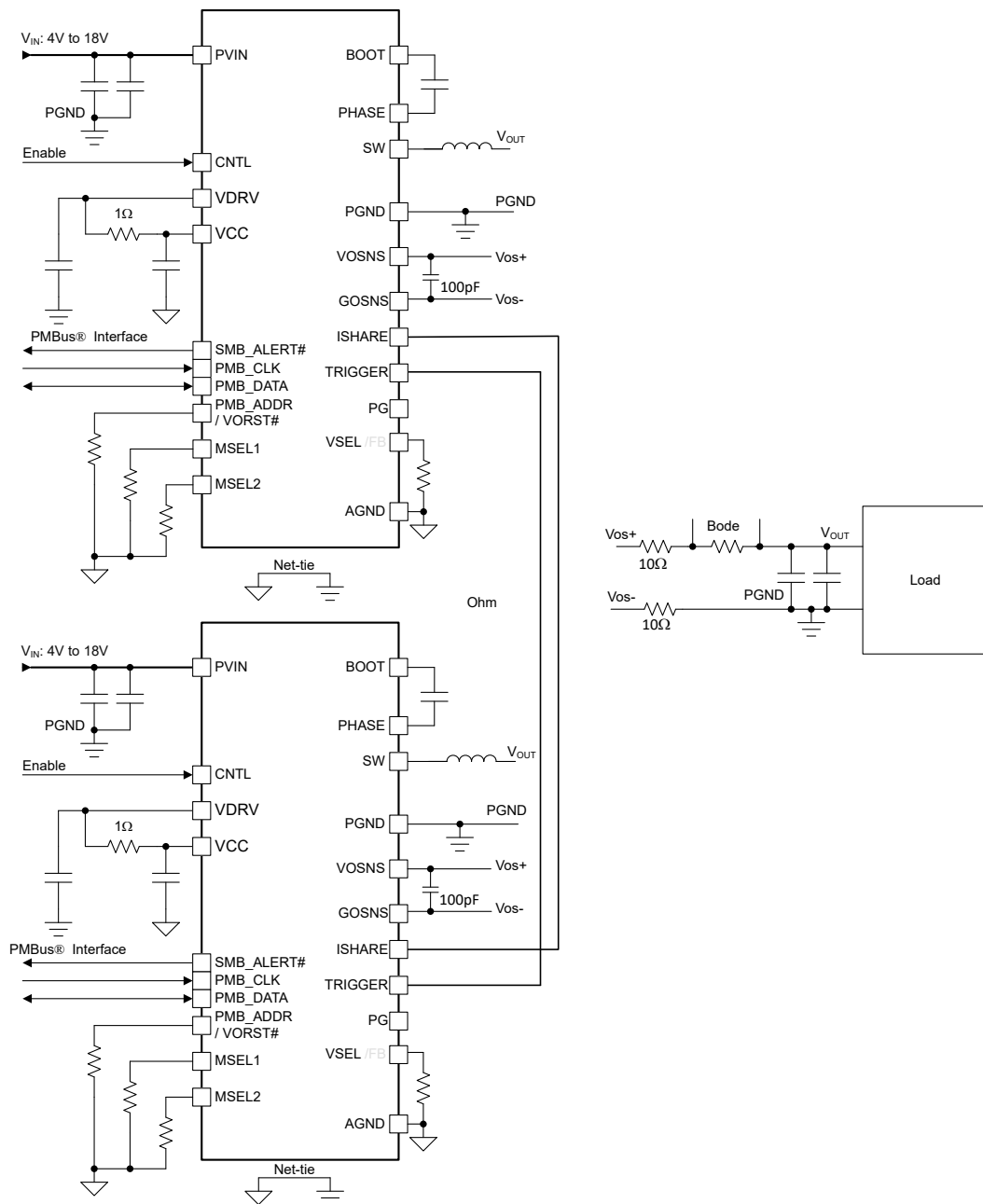
图 6-7. 两相配置内部分压器
