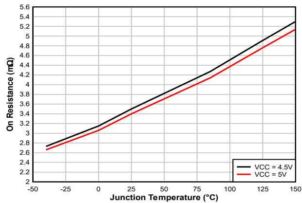
图 5-5. 高侧 MOSFET 导通电阻 ( R_{DS(on)} ) 与结温间的关系
