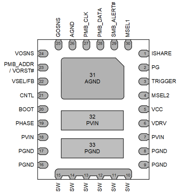
图 4-2. VBD 33 引脚 WQFN 封装 (底视图)
