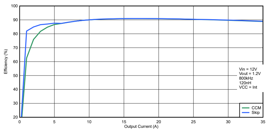
典型效率
