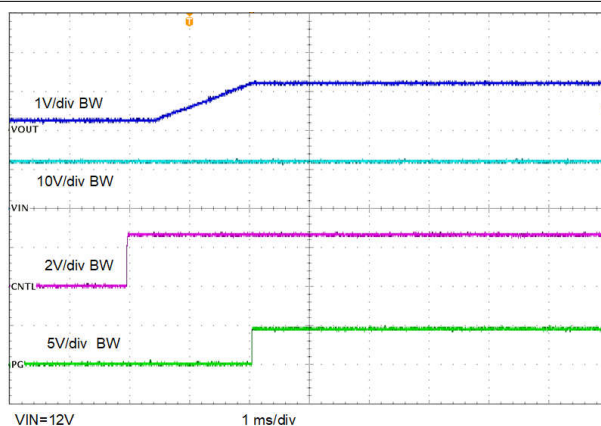
图 8-13. 具有预偏置输出的控制开启时启动波形
