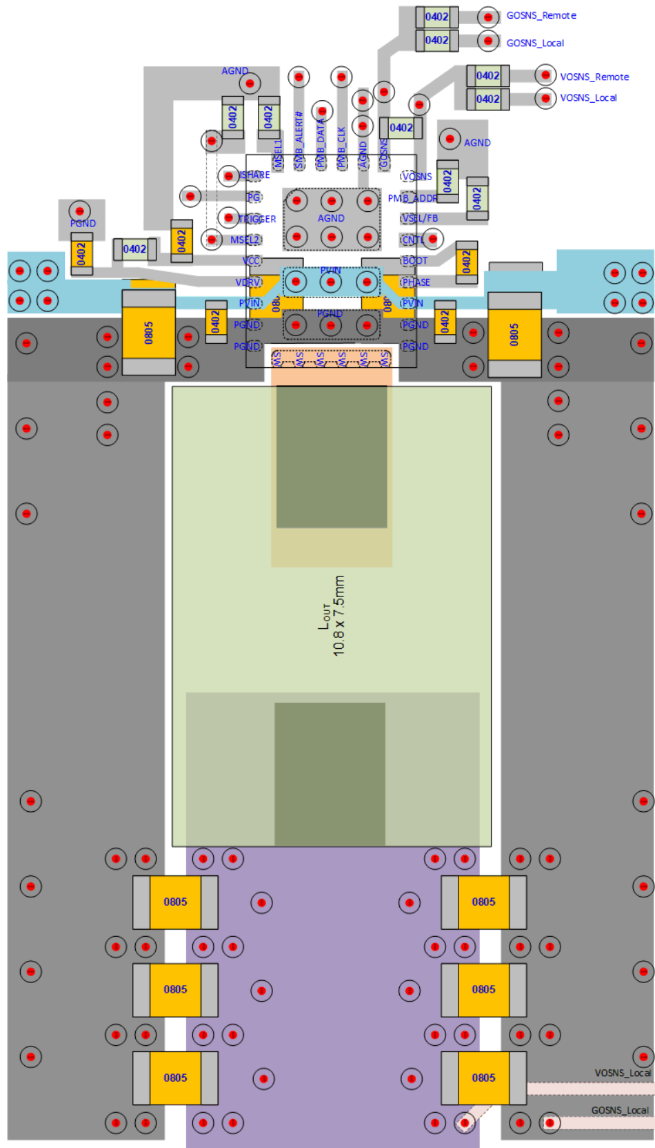
图 8-18. 布局建议
