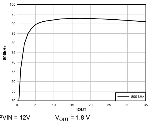
图 8-8. 效率, FCCM, 内部 LDO
