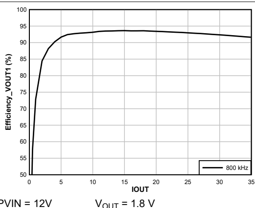
图 8-10. 效率, FCCM, 外部 5V 辅助电源
