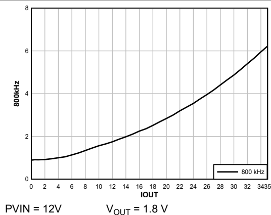
图 8-9. 功率耗散, FCCM, 内部 LDO
