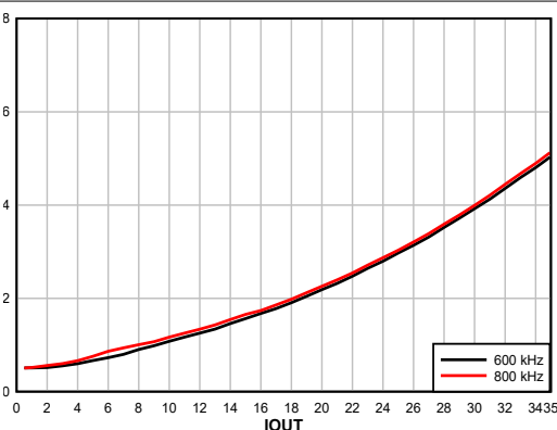
图 8-5. 功率耗散, FCCM, 内部 LDO
