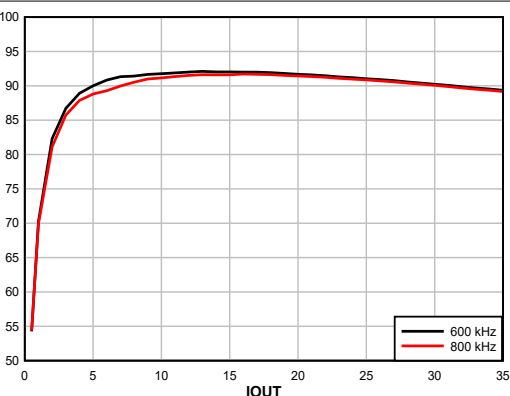
图 8-4. 效率, FCCM, 内部 LDO
