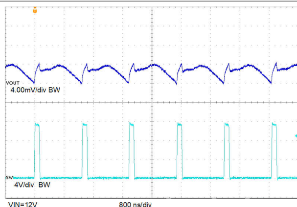
图 8-16. 输出电压纹波, 800kHz FCCM, 17.5A 负载
