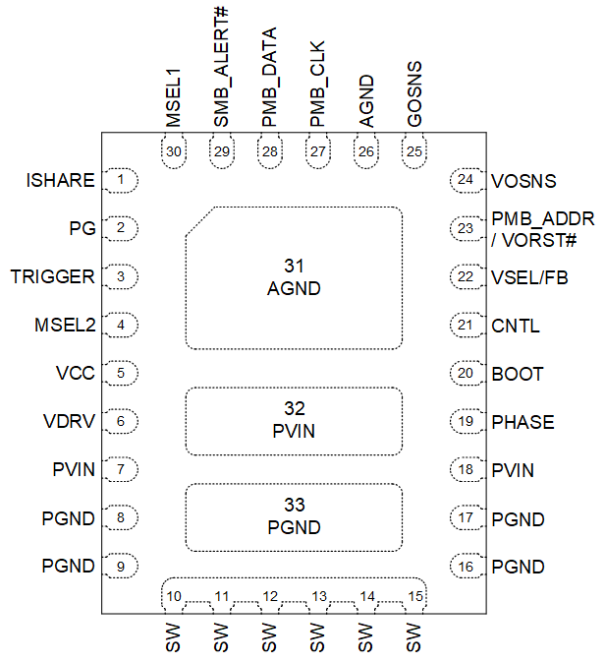
图 4-1. VBD 33 引脚 WQFN 封装 (顶视图)
