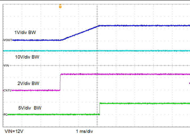
图 8-12. 控制开启时的启动, 0A 负载
