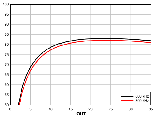
图 8-2. 效率, FCCM, 内部 LDO
