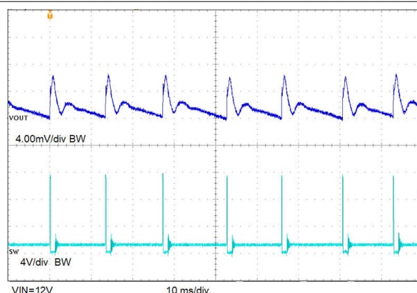
图 8-17. 输出电压纹波, 1.2V Vout, 800kHz DCM, 空载
