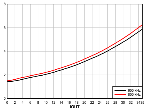
图 8-3. 功率耗散, FCCM, 内部 LDO
