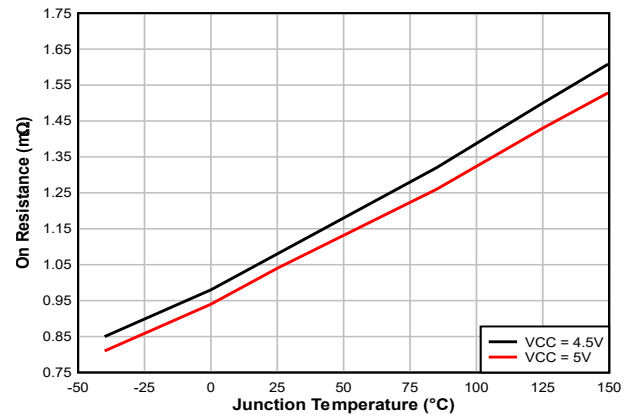
图 5-4. 低侧 MOSFET 导通电阻 ( R_{DS(on)} ) 与结温间的关系
