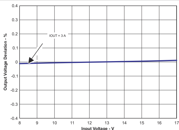
图 8-9. Line Regulation
