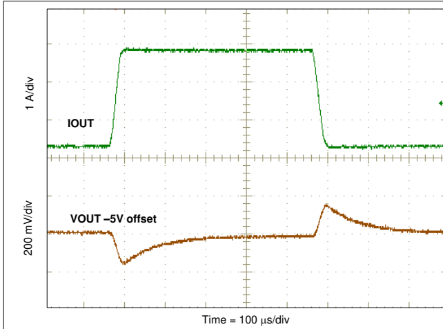
图 8-6. Load Transient
