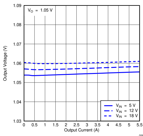
图 6-4. 1.05-V Output Voltage vs Output Current
