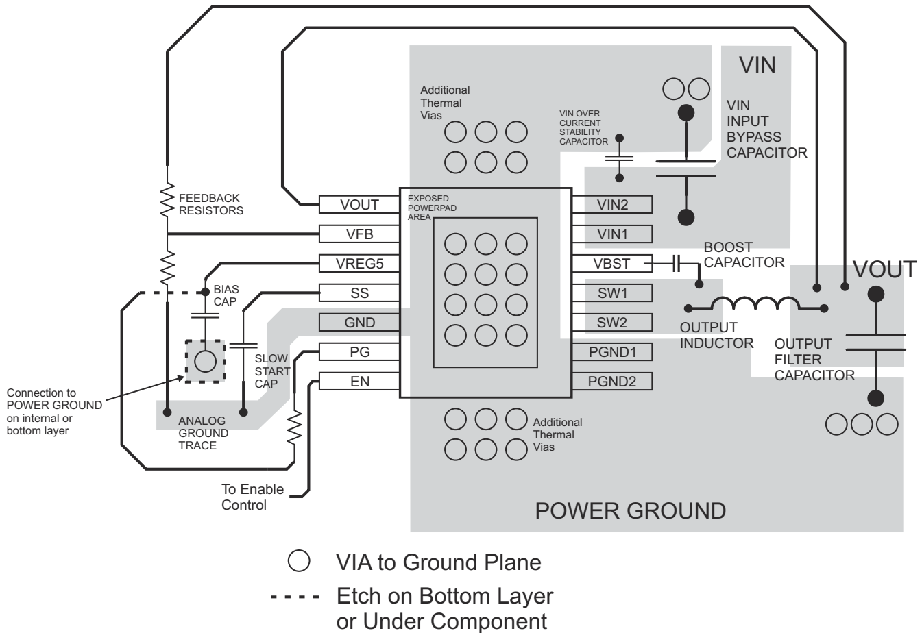
图 10-1. PCB Layout
