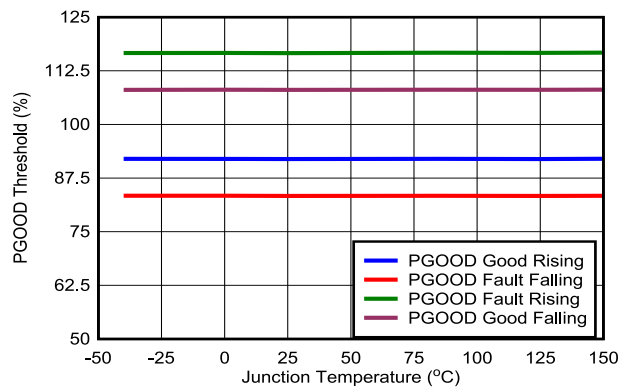
图 5-9. PG 阈值
