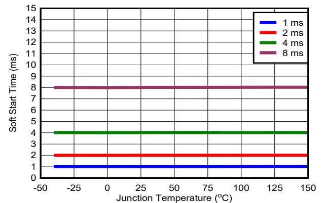
图 5-12. 软启动
