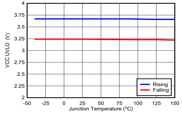
图 5-8. V_{CC} UVLO
