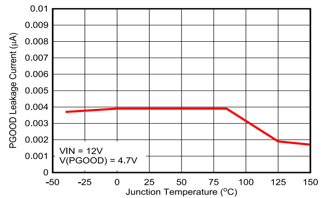
图 5-10. PG 漏电流
