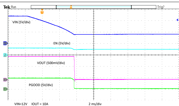
图 7-15. VIN 关断
