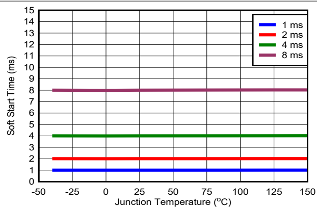
图 5-12. 软启动
