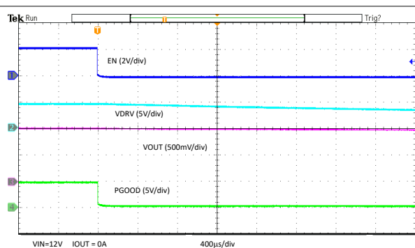
图 7-11. EN 关断
