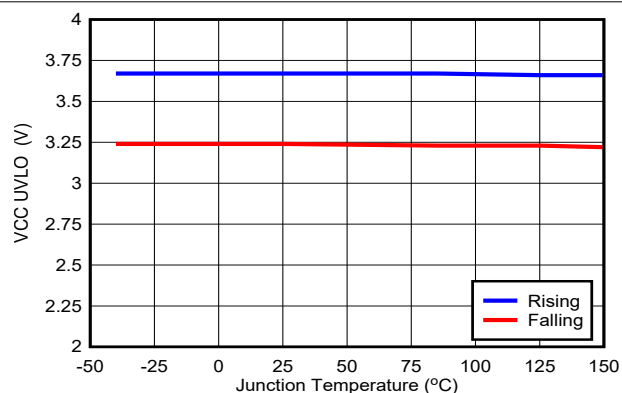
图 5-8. V_{CC} UVLO
