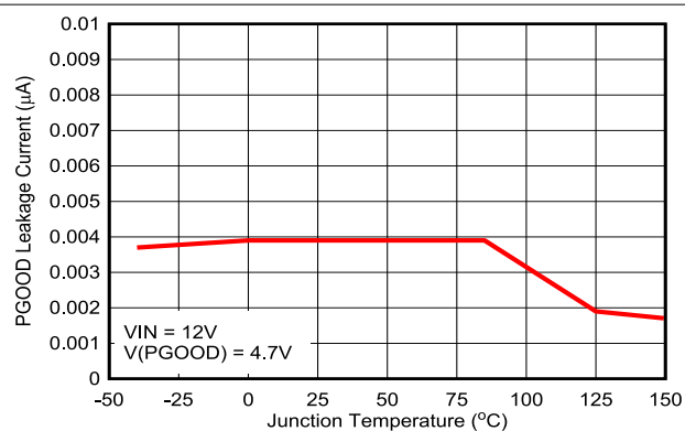
图 5-10. PG 漏电流
