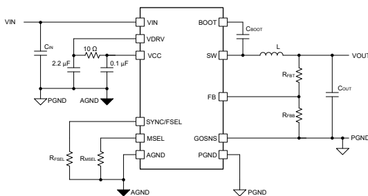
TPS543A26T 简化版应用
