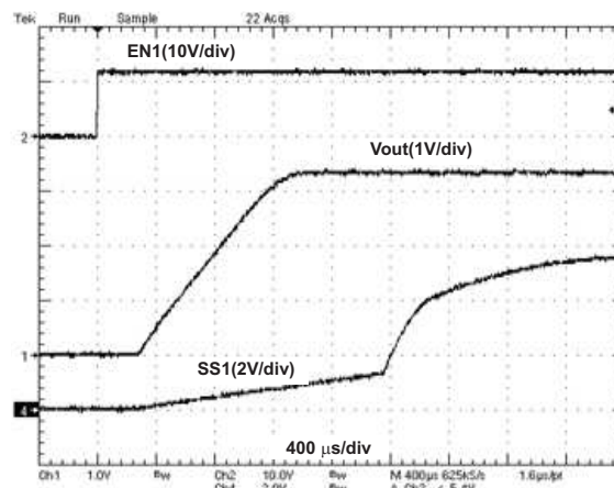
Figure 10. V_{O1}=3.3\text{V} , SoftStart
