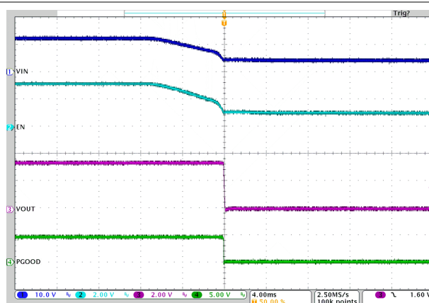
图 8-11. EN Shutdown
