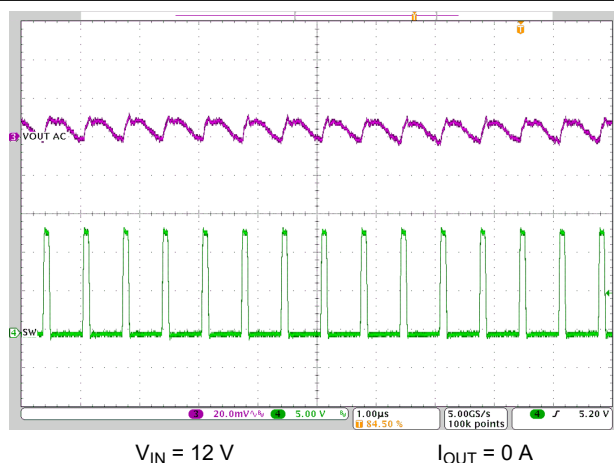
图 8-27. Output Ripple - No Load
