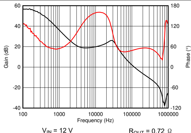
图 8-25. Bode Plot
