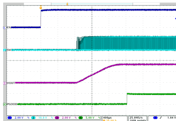
图 8-10. EN Startup - Measuring SW
