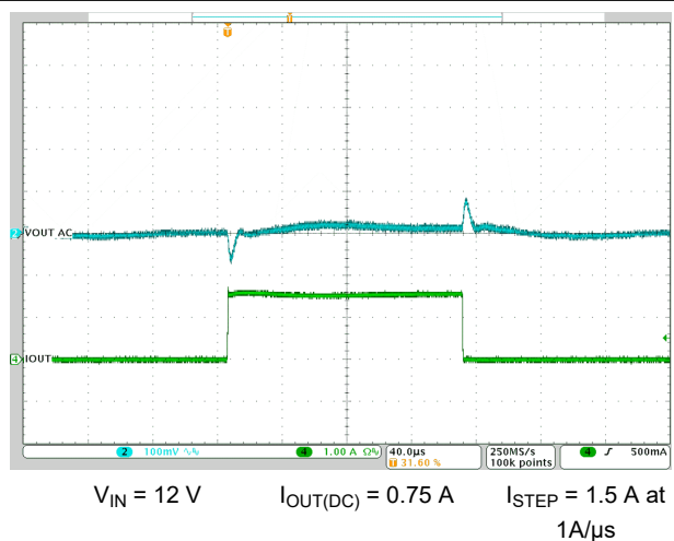
图 8-26. Load Transient
