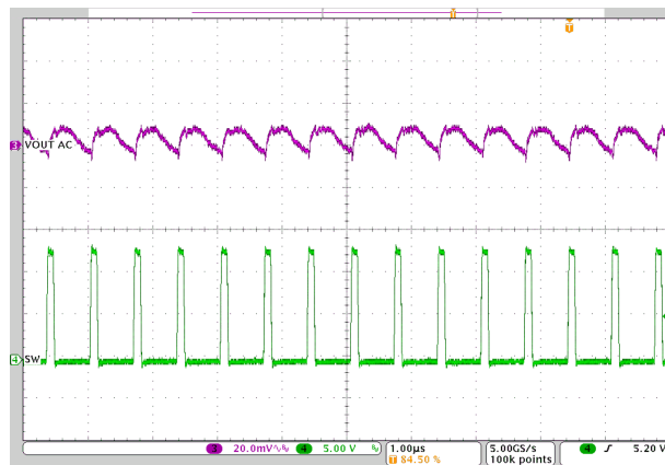
V_{IN} = 12\text{ V} I_{OUT} = 3\text{ A} 图 8-28. Output Ripple - 3-A Load
