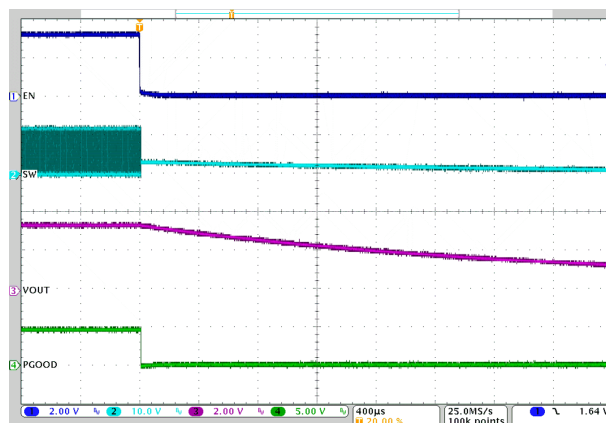
图 8-11. EN Shutdown
