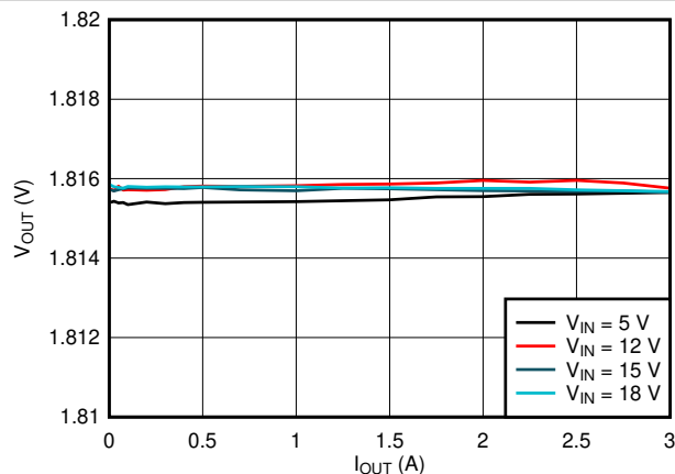
图 8-23. Load Regulation
