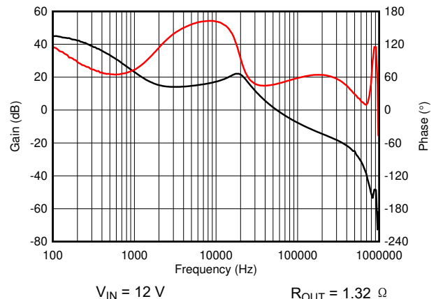
图 8-7. Bode Plot
