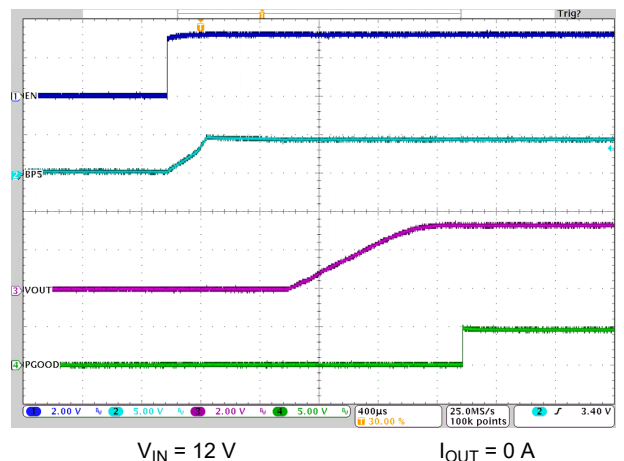
图 8-9. EN Start-up - Measuring BP5
