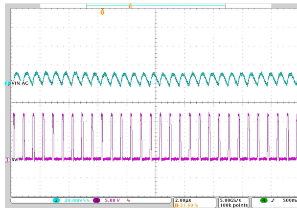
V_{IN} = 12\text{ V} I_{OUT} = 3\text{ A} 图 8-30. Input Ripple - 3-A Load
