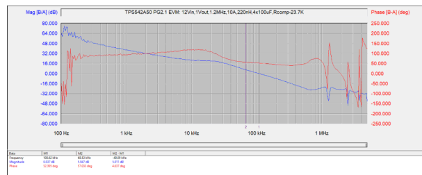
图 8-4. Bode Plot at 10-A Output Current
