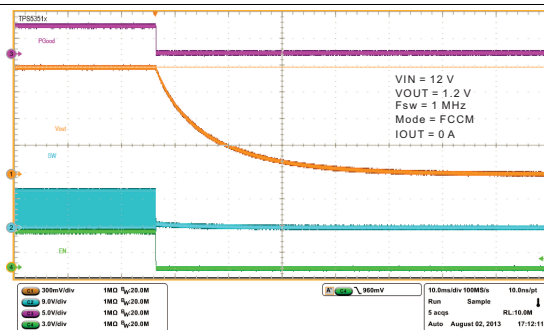
图 26. Shutdown Operation
