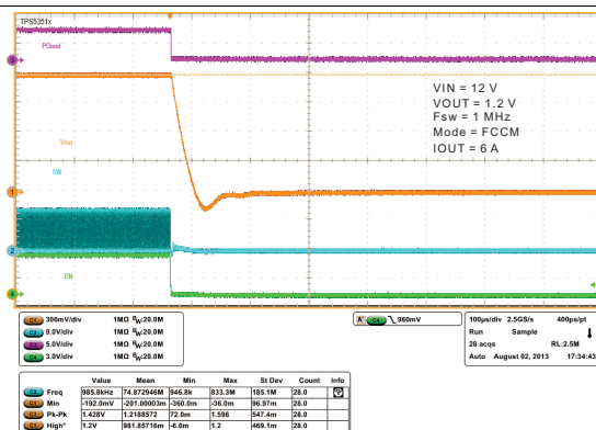
图 28. Shutdown Operation
