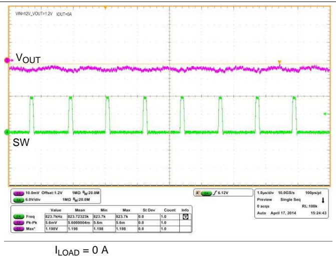
图 62. Output Voltage Ripple
