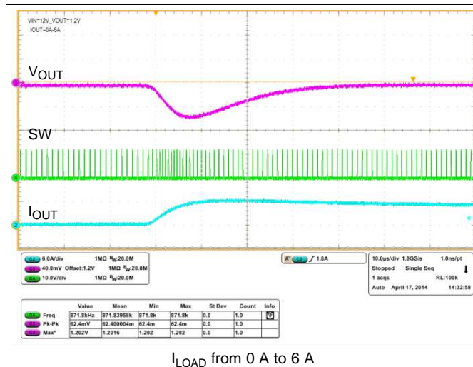
图 59. Load Transient
