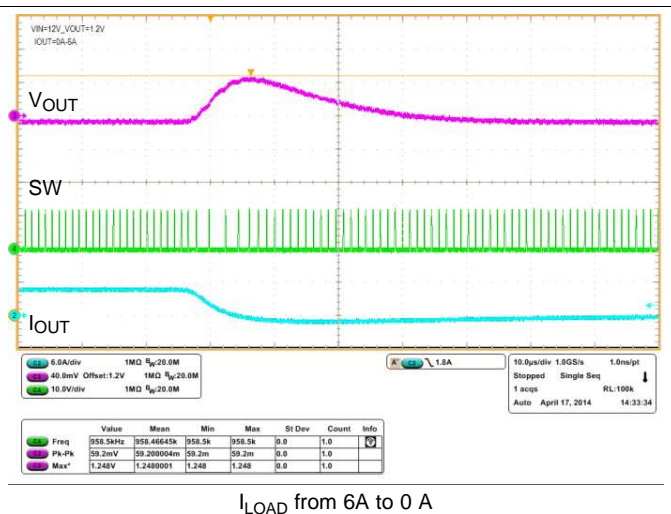
图 60. Load Transient
