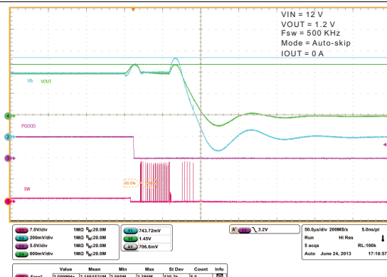
图 30. Overvoltage Protection
