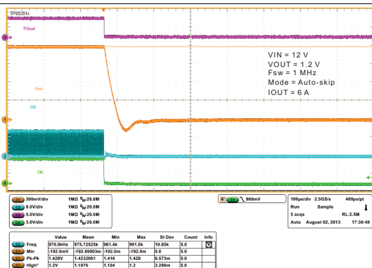
图 27. Shutdown Operation
