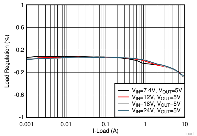
图 8-3. Load Regulation
