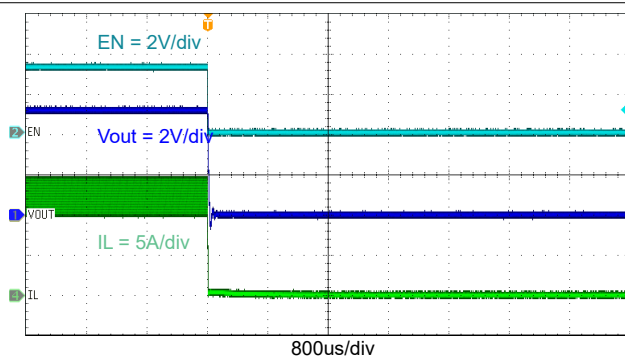
图 7-11. 通过 EN 关断, I_{OUT} = 12A
