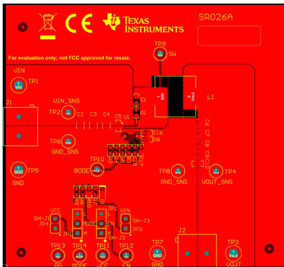
图 7-20. 顶面布局
