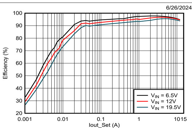
图 7-5. 效率曲线 ( OOA , F_{SW} = 920kHz )
