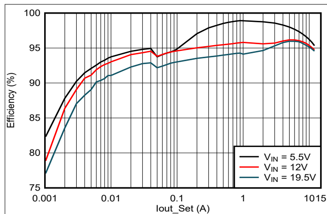
图 7-2. 效率曲线 (ECO)
