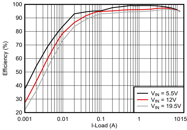
图 5-15. 效率与负载电流间的关系, 560kHz, OOA 模式
