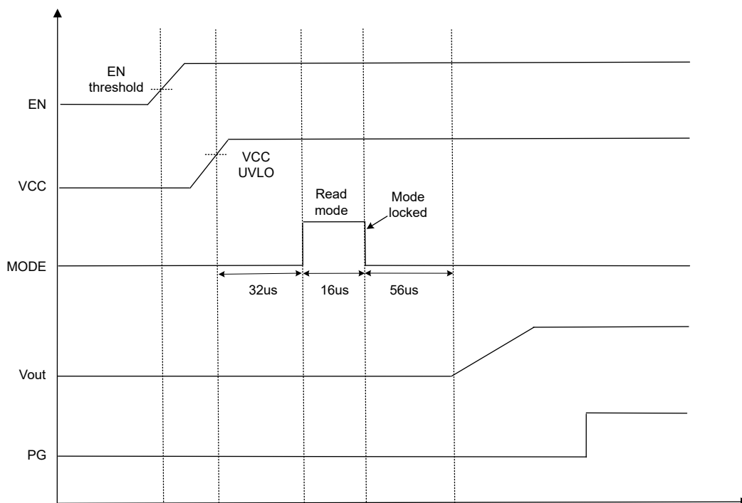
图 6-1. 上电序列
