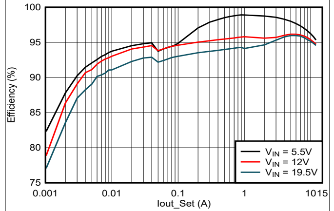
图 5-16. 效率与负载电流间的关系, 560kHz, Eco-mode
