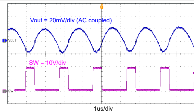
图 7-15. 输出电压纹波, I_{OUT} = 6A
