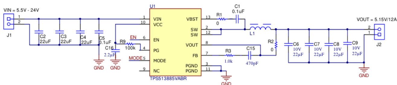
图 7-1. 5.15V、12A 参考设计
