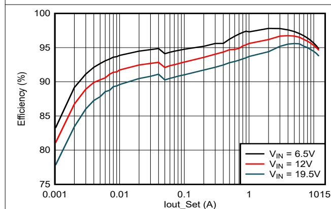
图 7-4. 效率曲线 ( ECO , F_{SW} = 920kHz )
