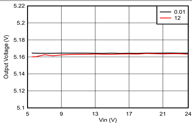
图 7-9. 线路调节, I_{OUT} = 0.01A/12A
