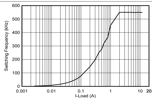
图 7-7. 开关频率与输出负载间的关系 (ECO)
