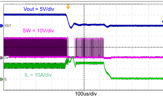
图 7-19. 正常运行至输出硬短路
