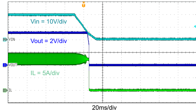
图 7-13. 相对于 V_{IN} 下降的关断, I_{OUT} = 5A
