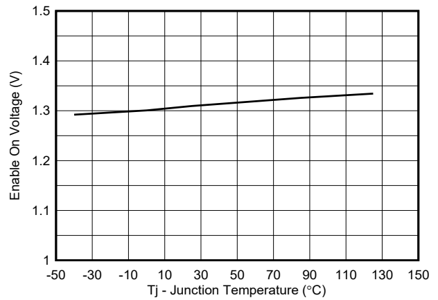
图 6-4. Enable On Voltage vs Temperature
