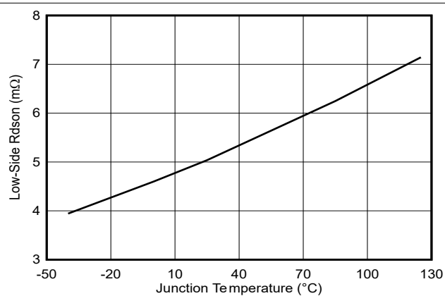
图 5-6. 低侧 R_{DS(on)} 与结温间的关系
