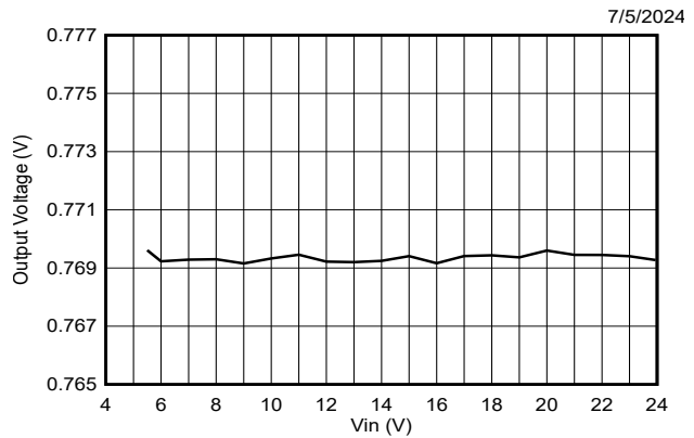
图 7-8. 线性调整率, I_{OUT} = 12A
