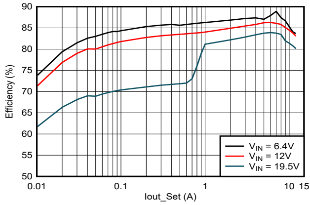
图 7-3. 效率曲线 ( V_{OUT} = 0.77V )
