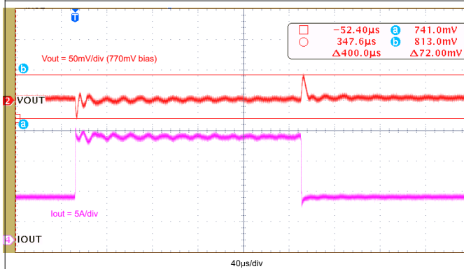
图 7-17. 瞬态响应, 7A 至 17A , 压摆率 = 10A/μs
