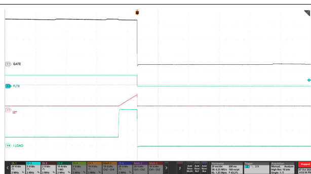
图 9-9. 6A 至 23A 负载阶跃下 TPS4812-Q1 EVM 基于 I²T 的过流响应
