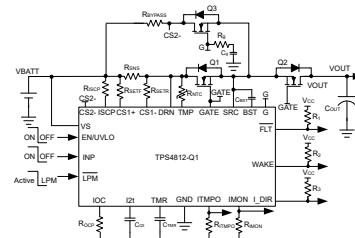
驱动 PAAT 负载、具有负载唤醒和大容量电容器充电功能的 TPS48120-Q1 应用电路
