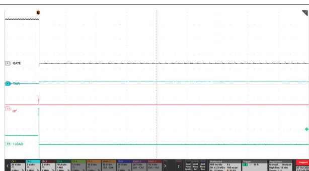
图 9-11. TPS4812-Q1 在 I²t 过流故障下的闭锁响应
