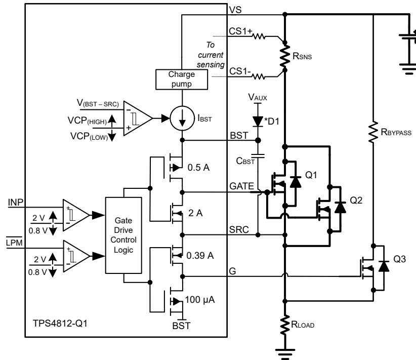
图 8-1. 栅极驱动器
