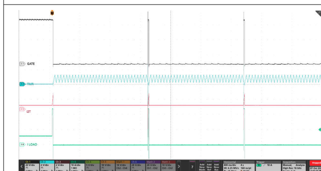
图 9-10. TPS4812-Q1 在 I²t 过流故障下的自动重试响应
