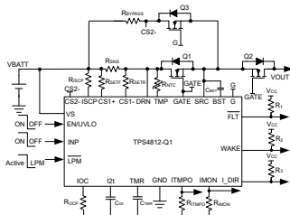
驱动 PAAT 负载、具有负载唤醒的 TPS48120-Q1 应用电路
