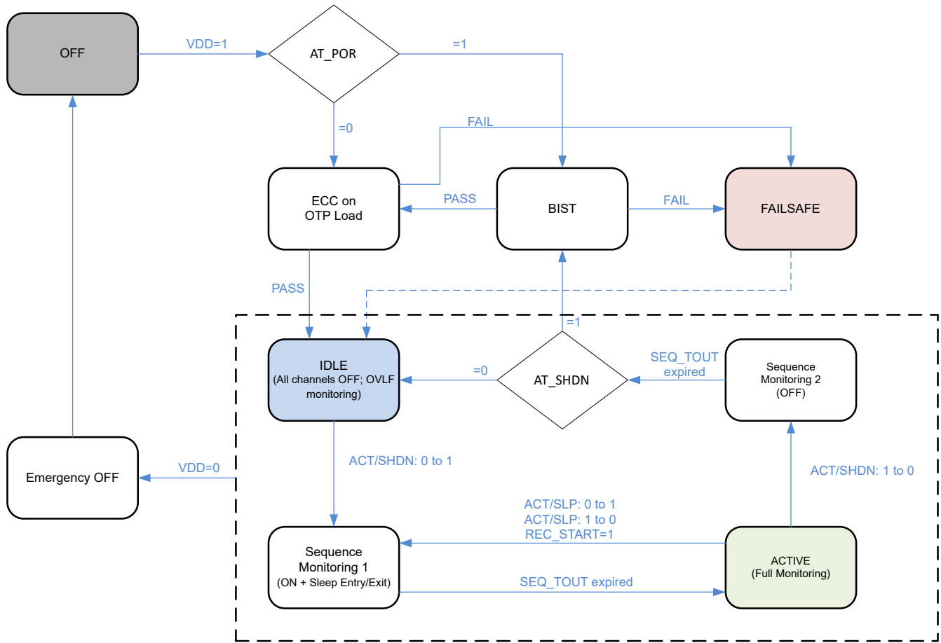
图 8-6. TPS389006 状态图
