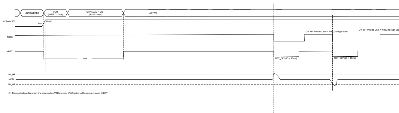
图 7-10. 电压故障的 NRST 时序图
