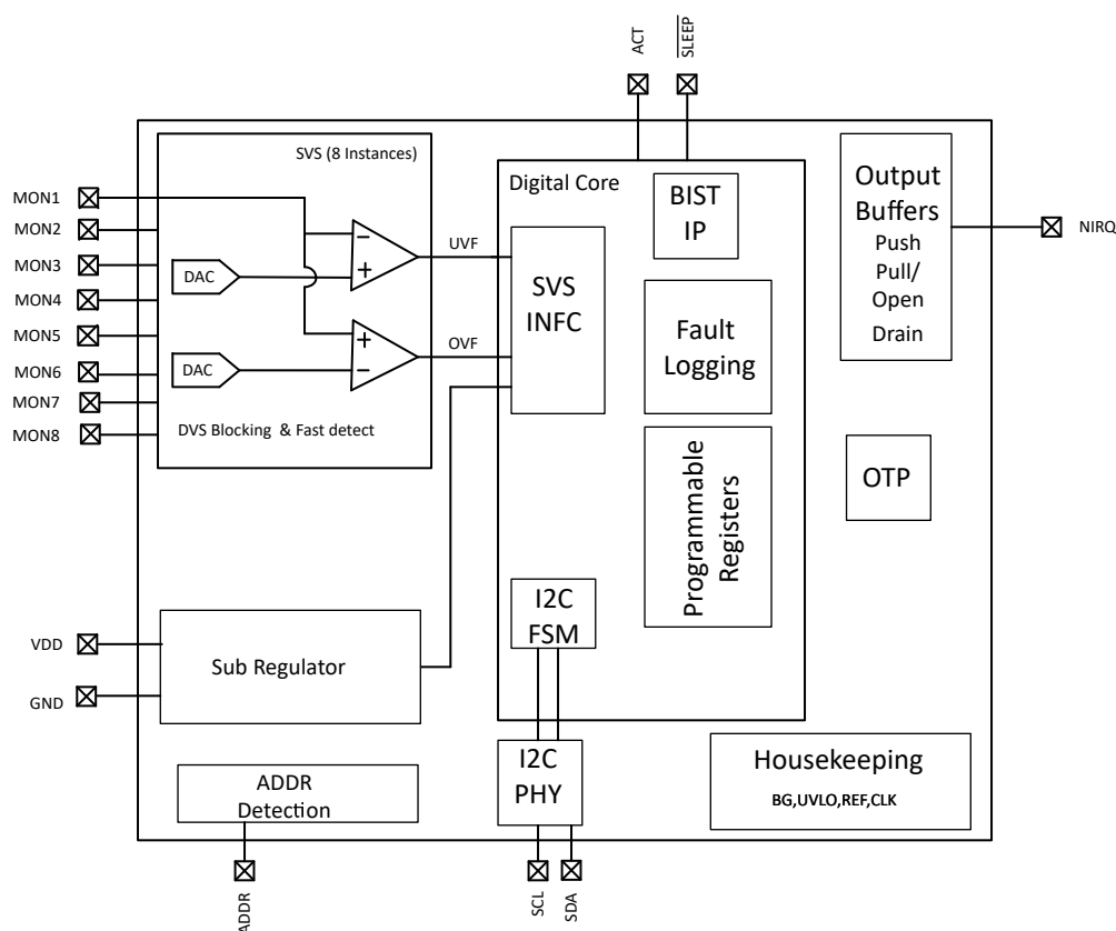
图 7-1. TPS38800-Q1 方框图
