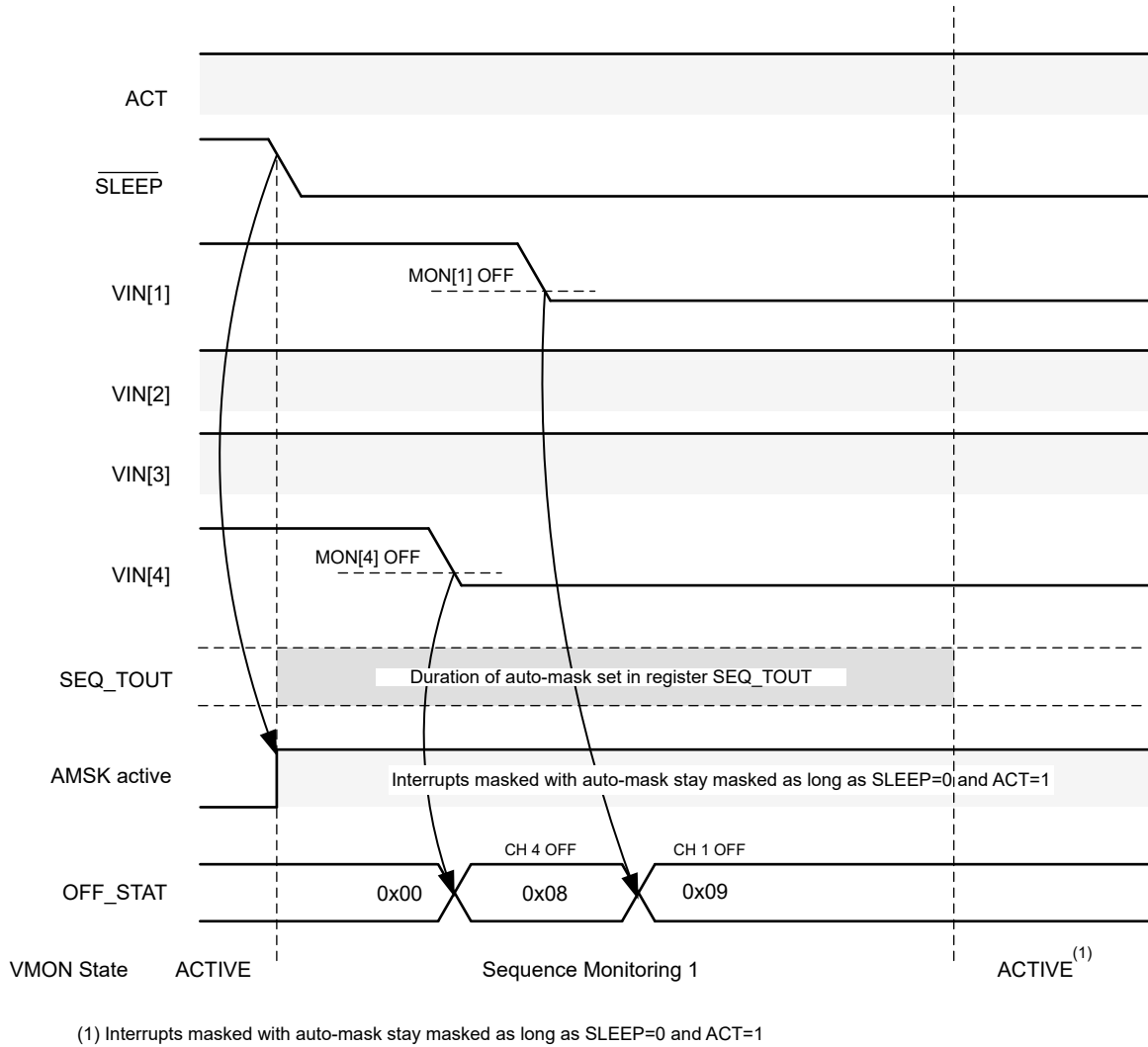
图 7-14. SLEEP 1→0 转换
