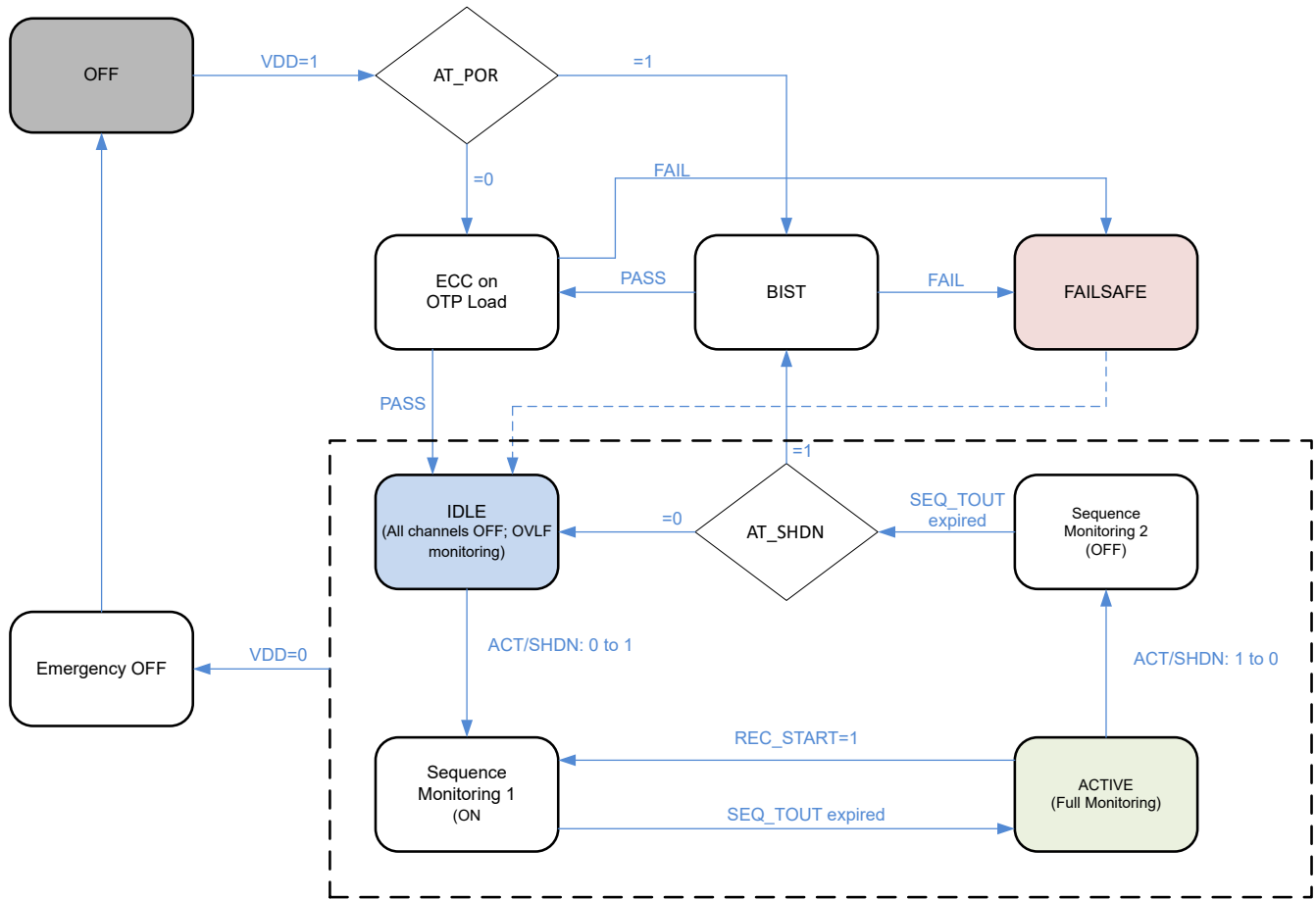
图 7-11. TPS38800-Q1/TPS388R0-Q1 状态图
