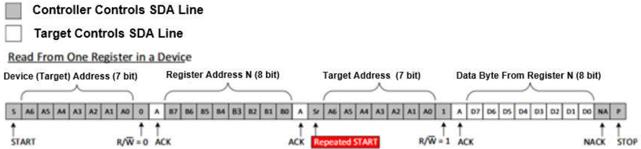
图 7-5. I 2 C 读取协议
