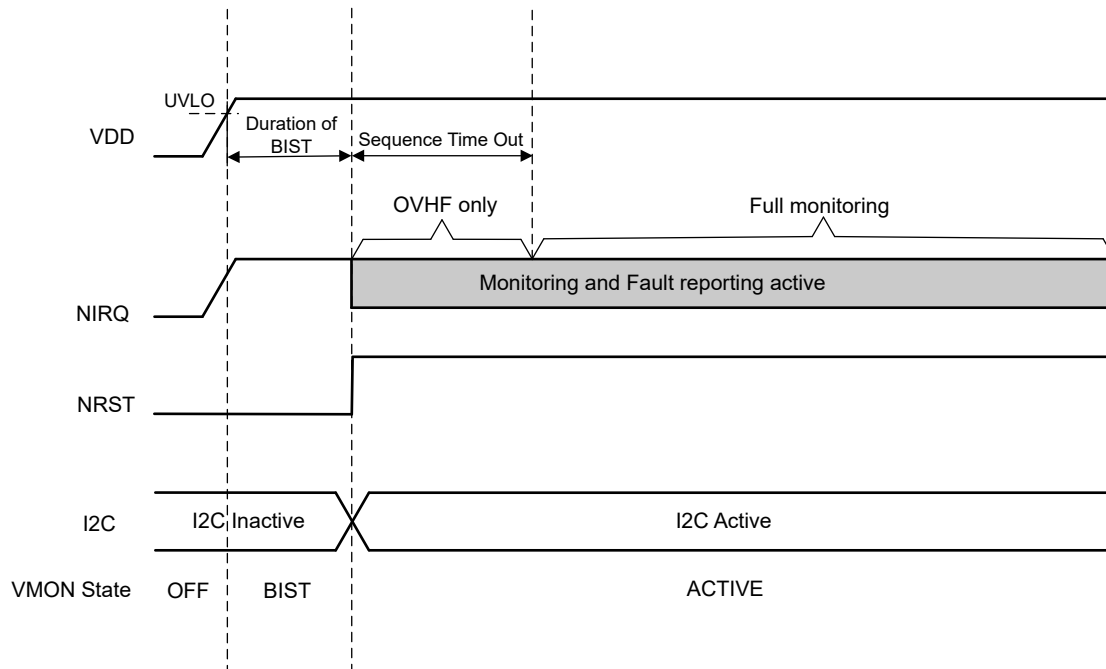
图 7-9. NRST 启动行为
