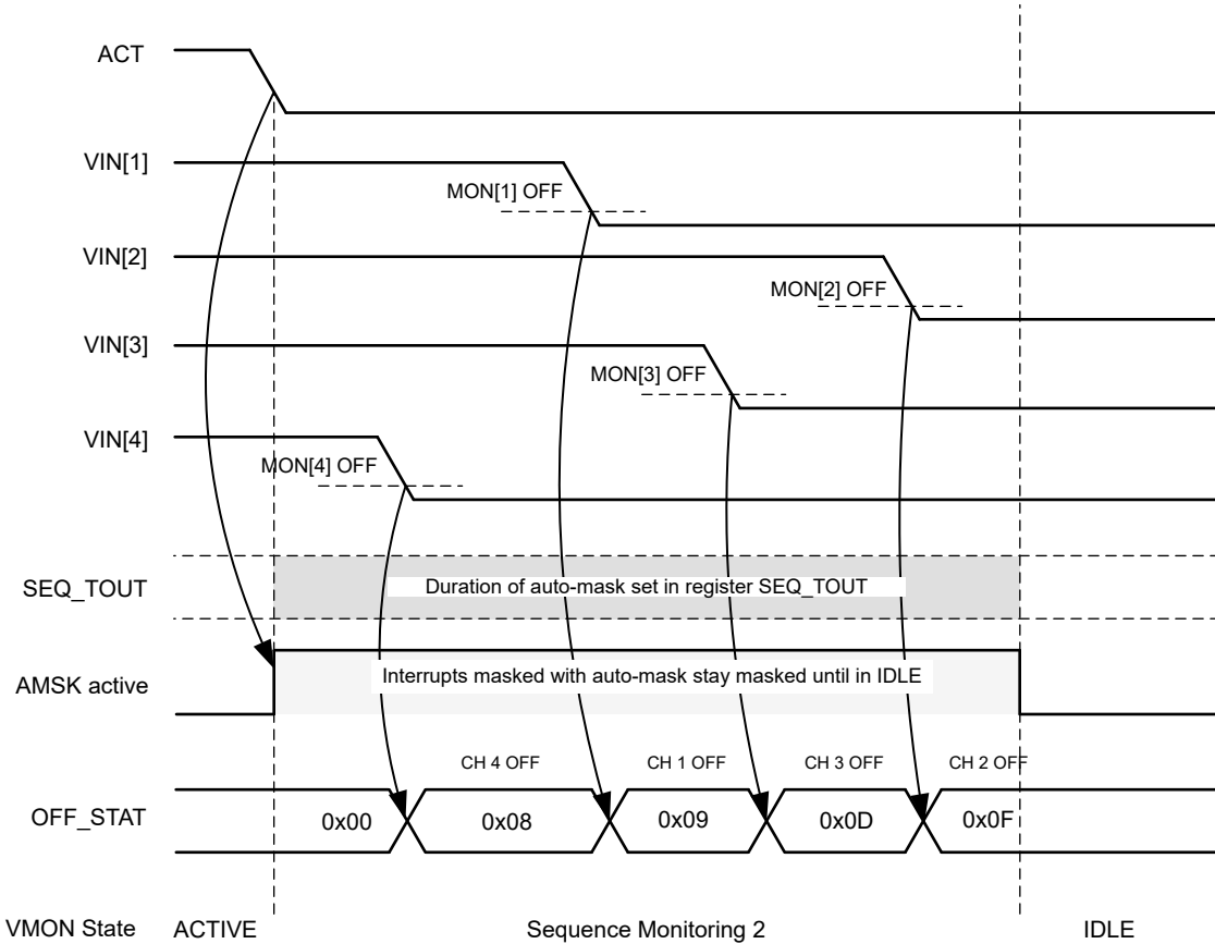
图 7-16. ACT 1→0 转换
