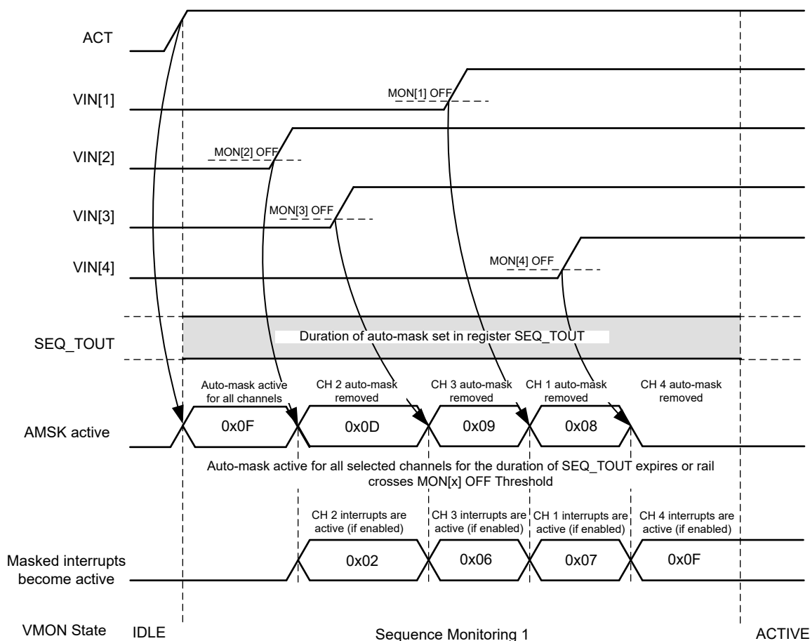
图 7-13. ACT 0→1 转换
