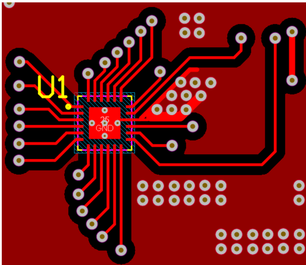
图 9-7. Recommended Layout
