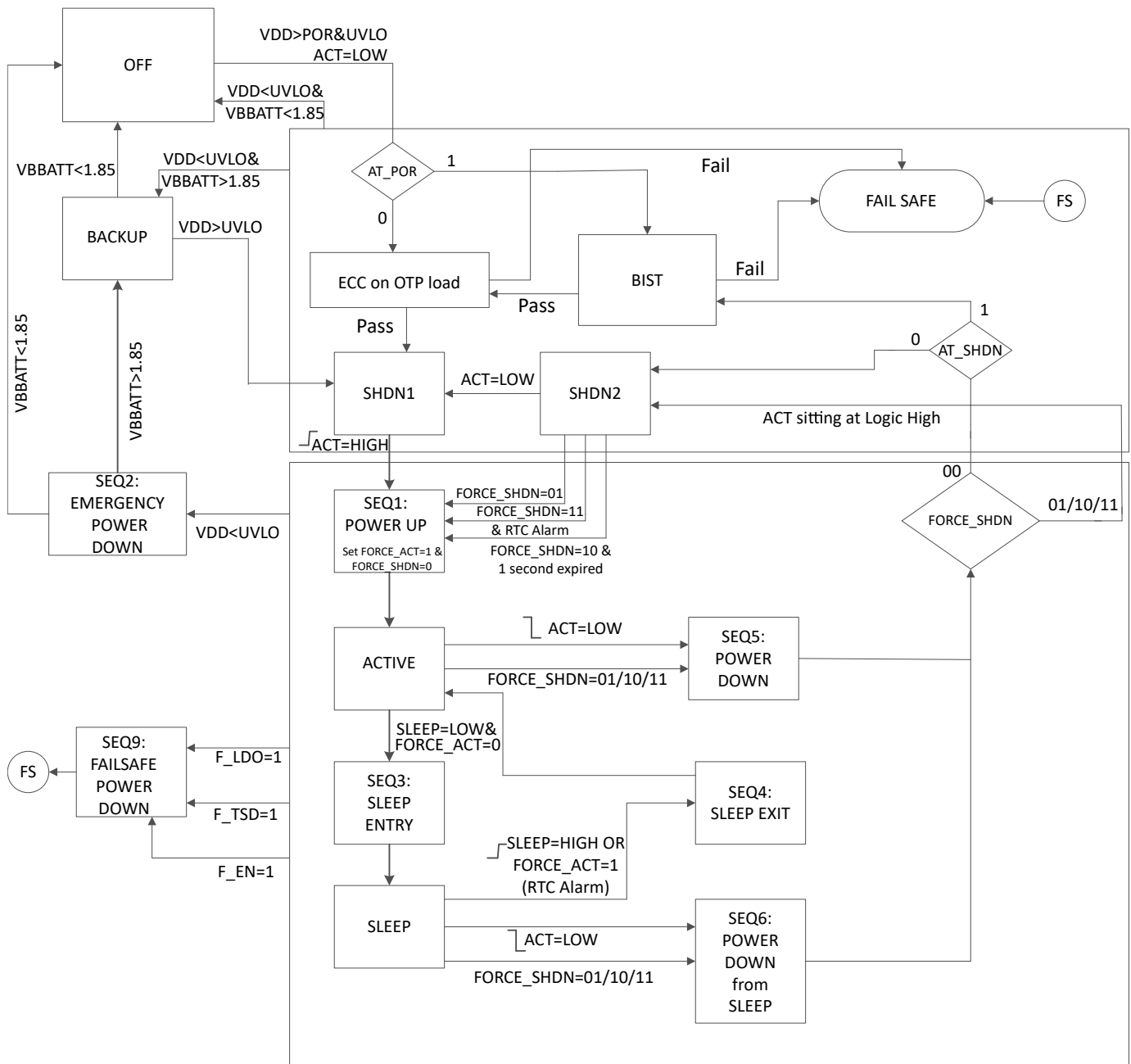
图 8-2. TPS38700 State Diagram
