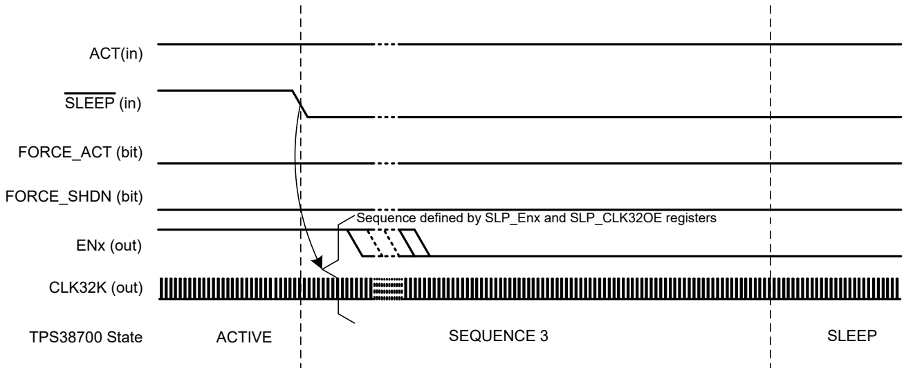
图 8-8. Sleep Entry
