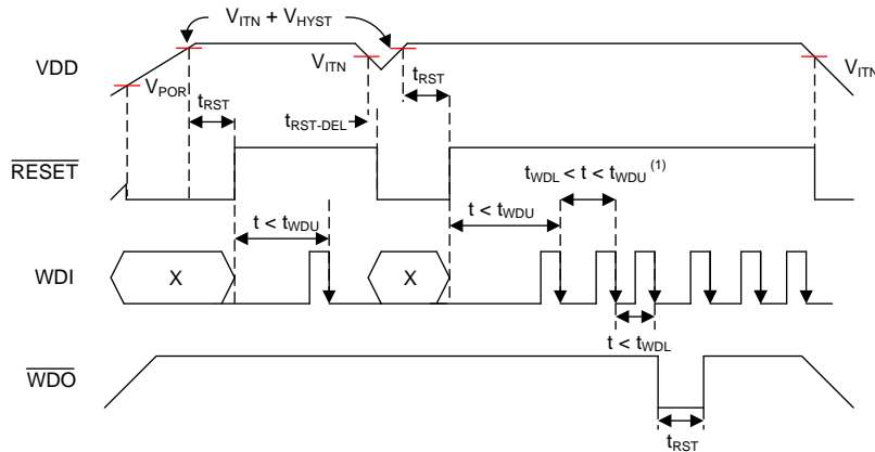
图 1. Timing Diagram
