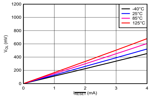
图 6-8. RESET 灌电流与 V_{\text{OL}} 间的关系 ( V_{DD} = 3.3\text{V} )
