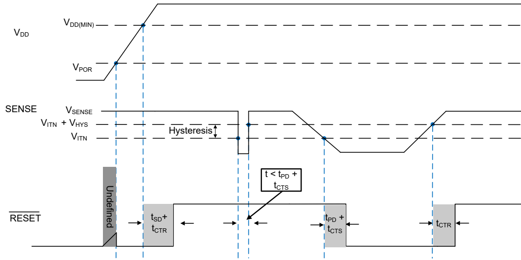
图 6-1. 欠压时序图
