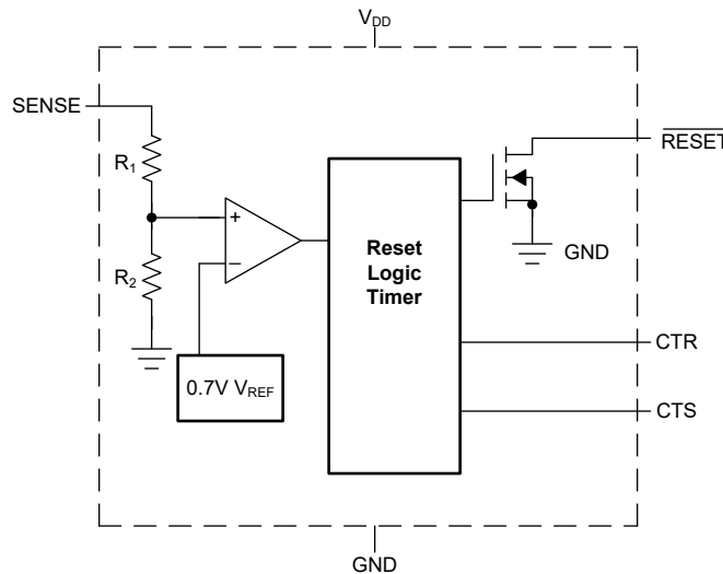
图 7-2. 欠压固定电压图
