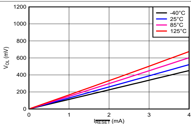
图 6-9. RESET 灌电流与 V_{\text{OL}} 间的关系 ( V_{\text{DD}} = 12\text{V} )
