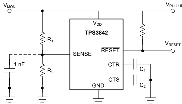
图 7-5. 使用 TPS3842A011DRLR 监控用户定义的阈值电压
