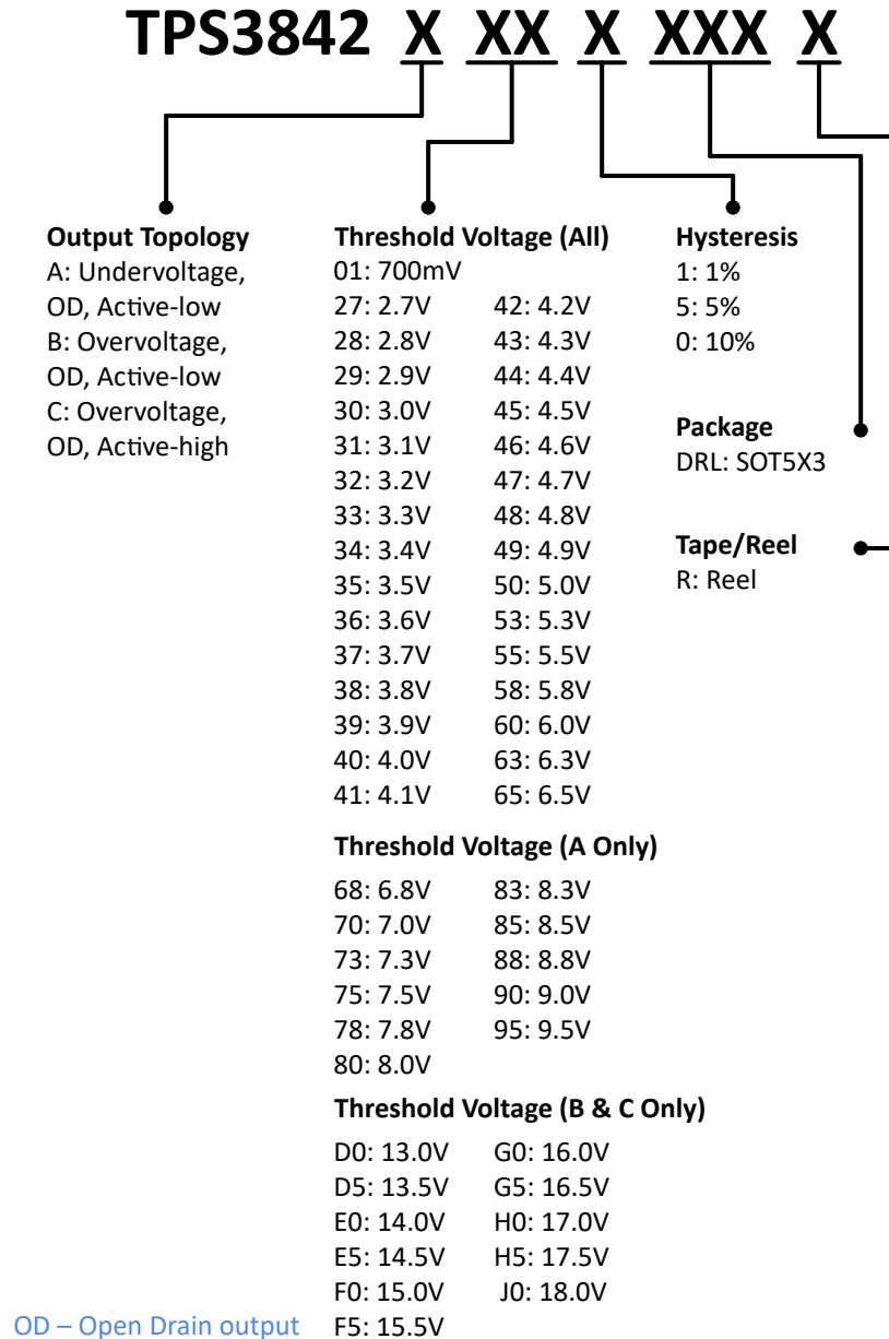
图 4-1. 器件命名约定
