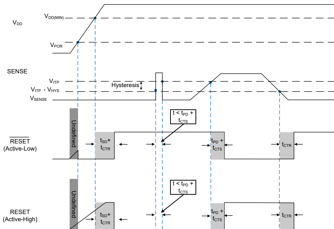
图 6-2. 过压时序图
