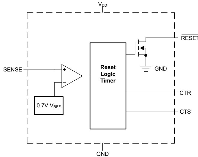
图 7-1. 欠压可调电压图
