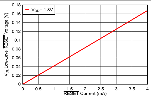
图 7-6. 低电平 RESE 电压与 RESE 电流间的关系
