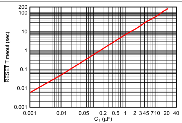
图 7-2. RESE 超时周期与 C_T 间的关系
