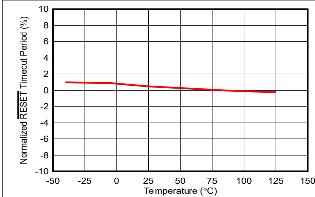
图 7-3. 标准化 RESE 超时周期与温度间的关系 ( C_T = 开路, C_T = V_{DD} , C_T = 任意)
