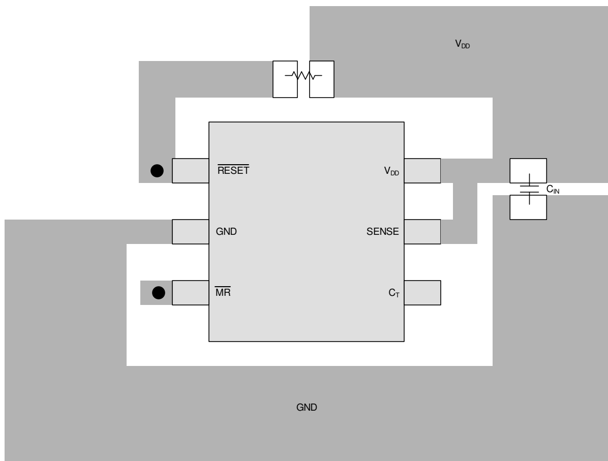
图 9-4. 20ms 延迟的布局示例
