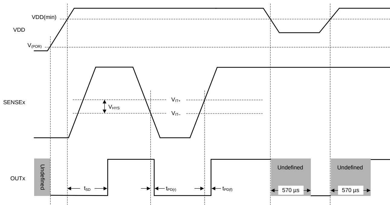
图 1. Timing Diagram
