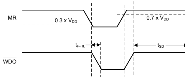
图 7-10. \overline{\text{MR}} 引脚响应
