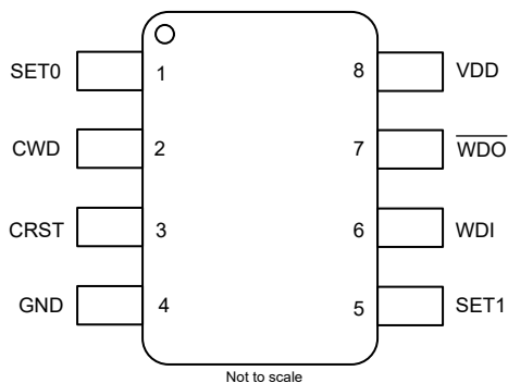
图 5-2. 引脚配置选项 B DDF 封装，8 引脚 SOT-23， TPS3435-Q1 顶视图
