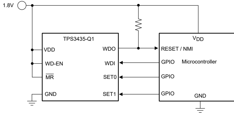
图 8-1. 微控制器看门狗监控电路
