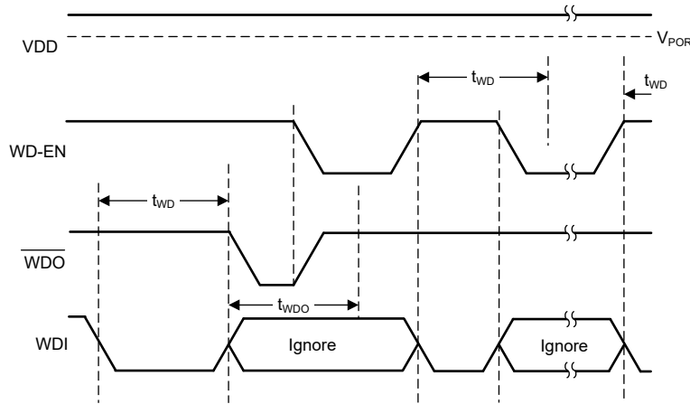
图 7-5. 看门狗启用 : WD-EN 引脚控制
