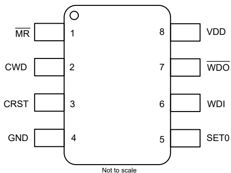
图 5-1. 引脚配置选项 A DDF 封装，8 引脚 SOT-23， TPS3435-Q1 顶视图
