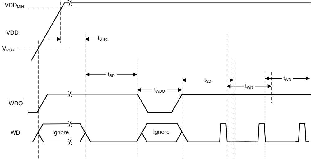
图 7-6. t_{SD} 帧行为
