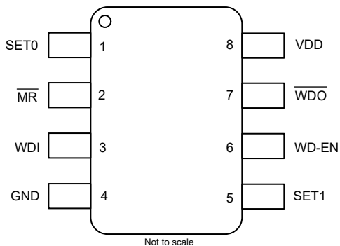
图 5-3. 引脚配置选项 C DDF 封装，8 引脚 SOT-23， TPS3435-Q1 顶视图
