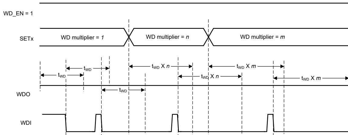
图 7-7. 具有 SETx 引脚状态的看门狗行为
