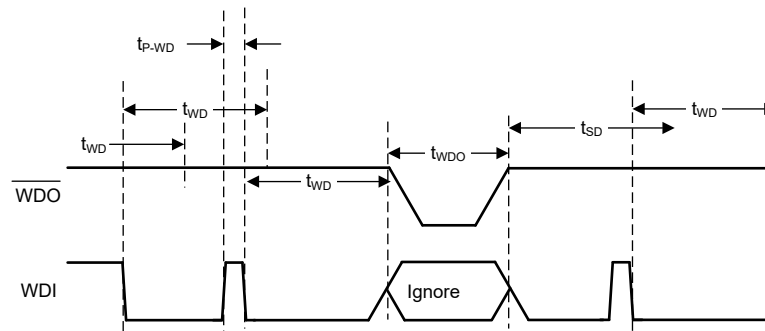
图 7-4. 超时看门狗计时器运行情况
