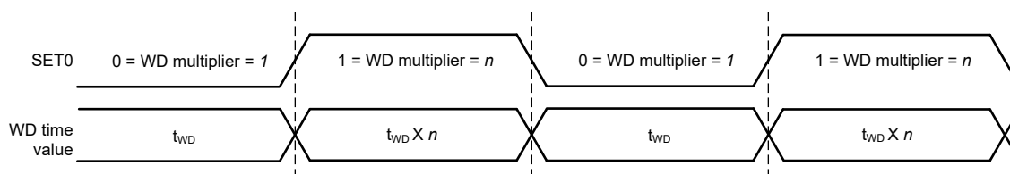
图 7-8. 具有 2 个 SET 引脚的看门狗运行情况
