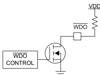
图 8-2. 开漏 \overline{WDO} 配置
