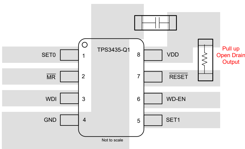
图 8-3. 引脚排列 C 的典型布局 - TPS3435-Q1
