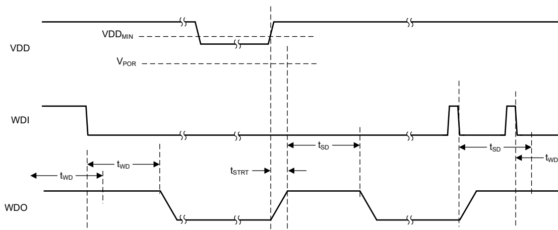
图 7-11. 输出锁存器时序行为
