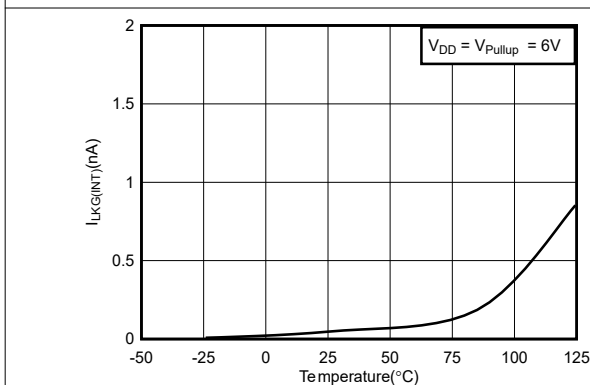
图 6-9. INT 漏电流与温度间的关系
