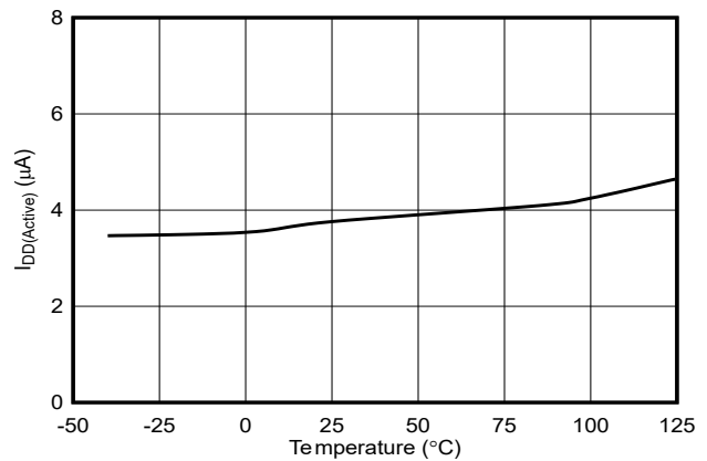
图 6-6. 有效电流与温度间的关系 (低电平有效按钮输入)
