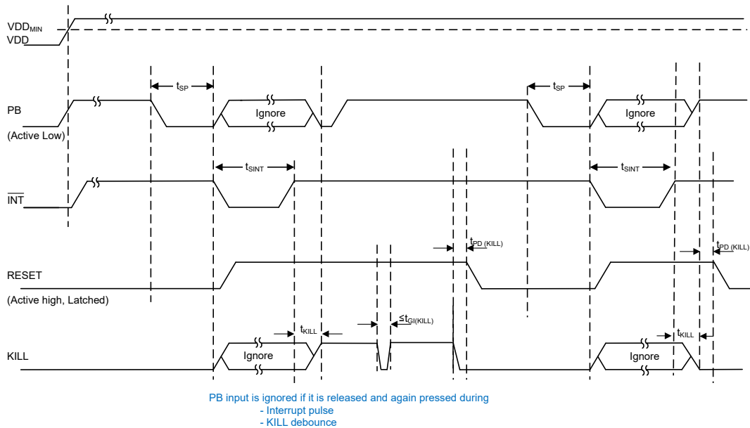
图 6-4. 时序图：KILL
