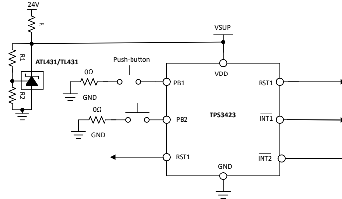
图 8-3. 通过 ATL431 提供高电压支持
