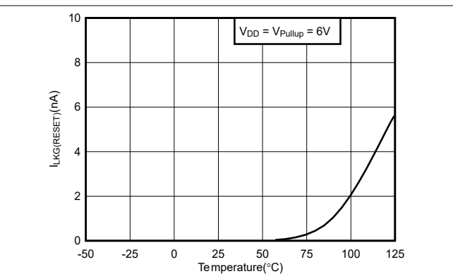
图 6-10. 开漏 RESET 漏电流与温度间的关系
