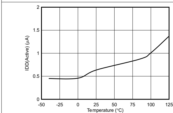
图 6-7. 有效电流与温度间的关系 (高电平有效按钮输入)
