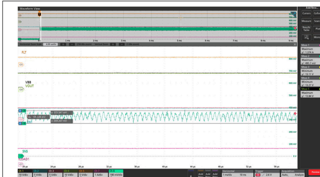
图 8-10. SNS 引脚无 C_{SNS} 时的纹波 ( V_{BS} = 13.5V , I_{LIM} = \text{开路} , R_L = 10\Omega , R_{SNS} = 1k\Omega , T_A = 25^\circ C )
