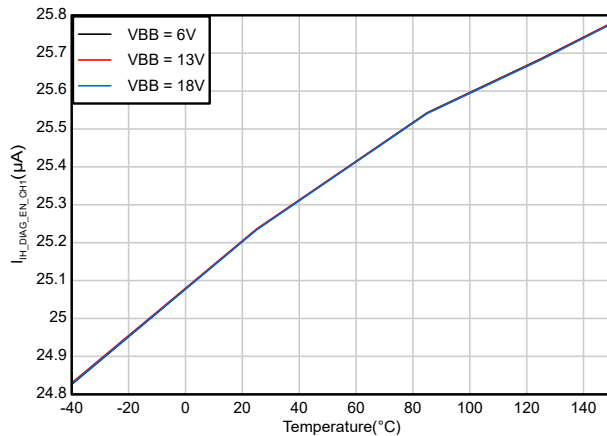
图 6-29. 通道 1 的 DIAG_EN 输入电流高电平与温度间的关系
