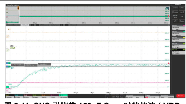
图 8-11. SNS 引脚带 150pF C_{SNS} 时的纹波 ( V_{BS} = 13.5V , I_{LIM} = \text{开路} , R_L = 10\Omega , R_{SNS} = 1k\Omega , T_A = 25^\circ C )
