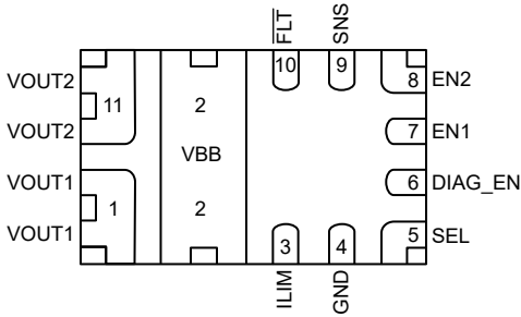
图 5-1. VAH 封装 TPS2HC16-Q1 顶视图
