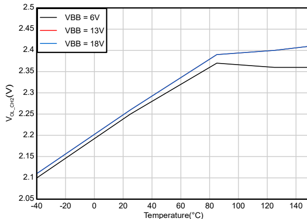
图 6-32. 通道 2 的开路负载检测电压 ( V_{OL} ) 与温度间的关系
