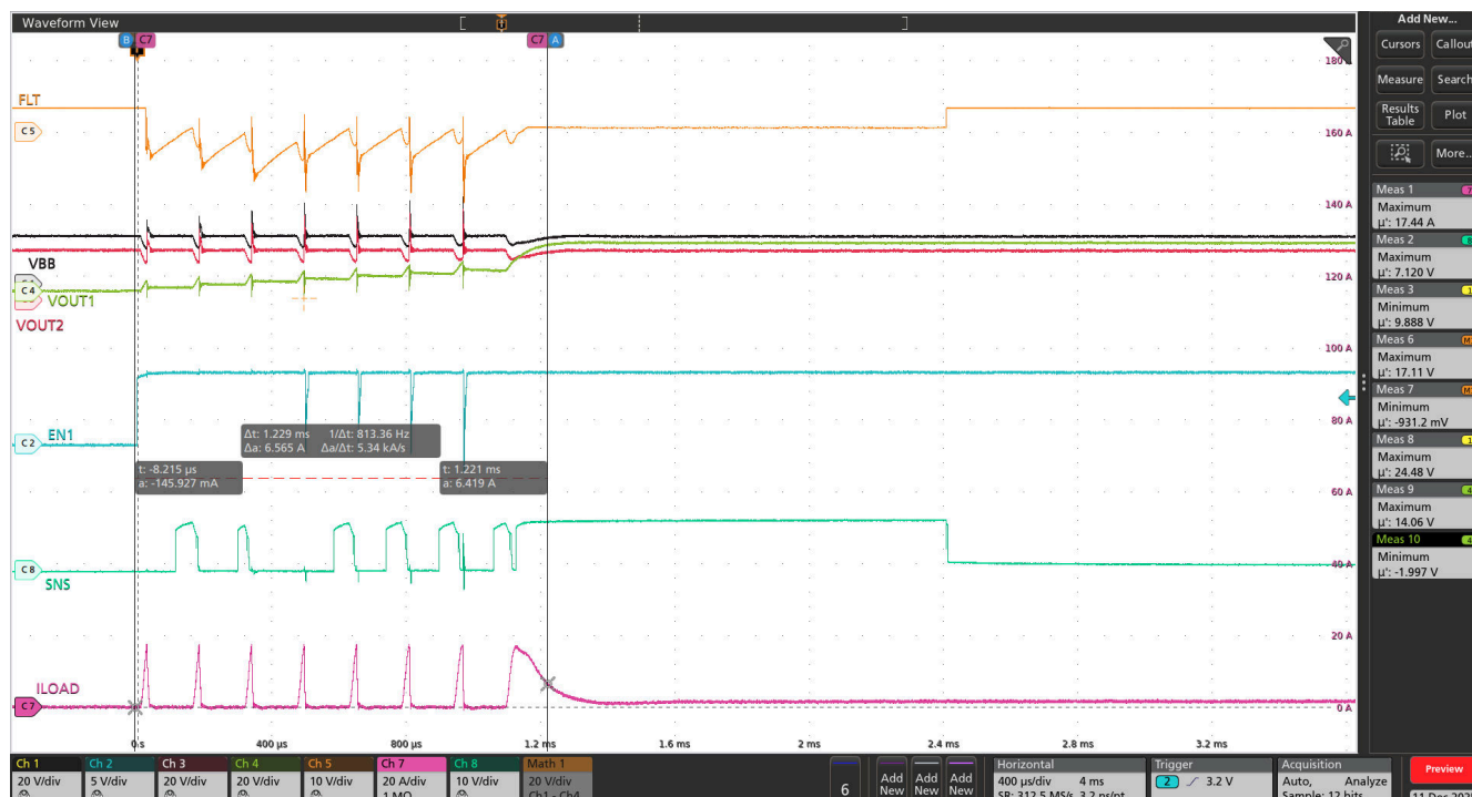
图 8-29. 使用 TPS2HC16-Q1 器件的通道 1 在 13.5V VBB、ILIM 引脚对地短路和 125°C 环境温度下实现 220 \mu F 容性负载充电（通道 2 上无负载）
