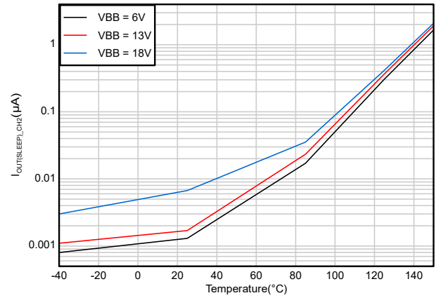
图 6-4. 通道 2 输出泄漏电流 ( I_{\text{OUT(SLEEP)}}_{\text{CH2}} ) 与温度间的关系
