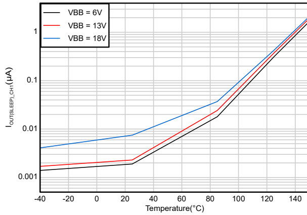
图 6-3. 通道 1 输出泄漏电流 ( I_{\text{OUT(SLEEP)}}_{\text{CH1}} ) 与温度间的关系
