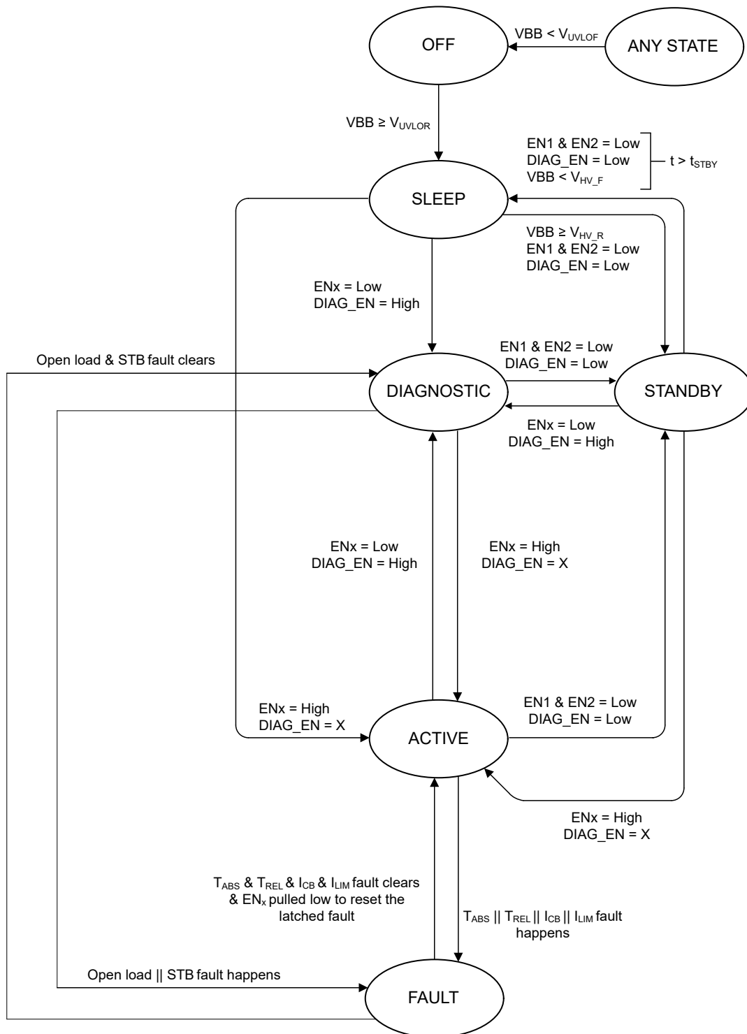
图 8-43. 状态图
