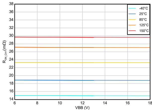
图 6-5. 通道 1 的导通电阻 ( R_{\text{ON}} ) 与 VBB 间的关系
