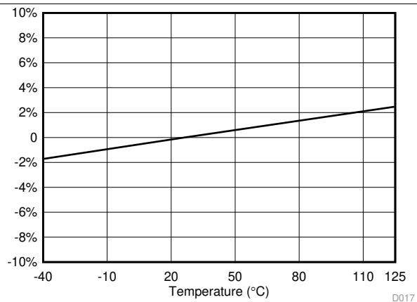
图 16. I_{OL,on}
