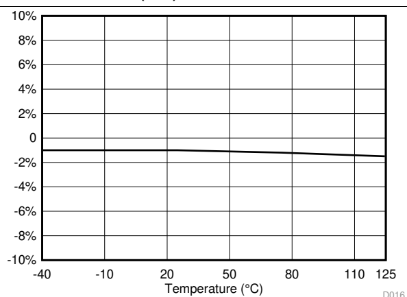
图 18. K_{(IMON)} at I_{OUT} = 25\text{ mA} , V_{IN} = 24\text{ V}
