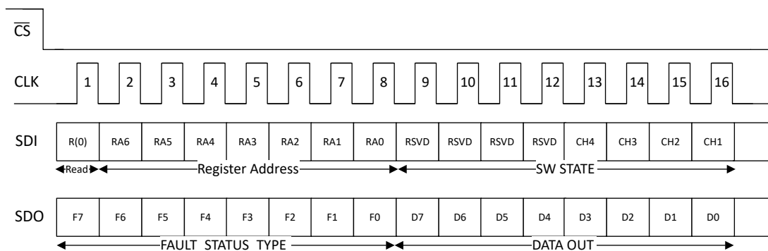
图 8-11. 16-bit Read, DSPI=1, D24BIT=0, CRC_EN=0
