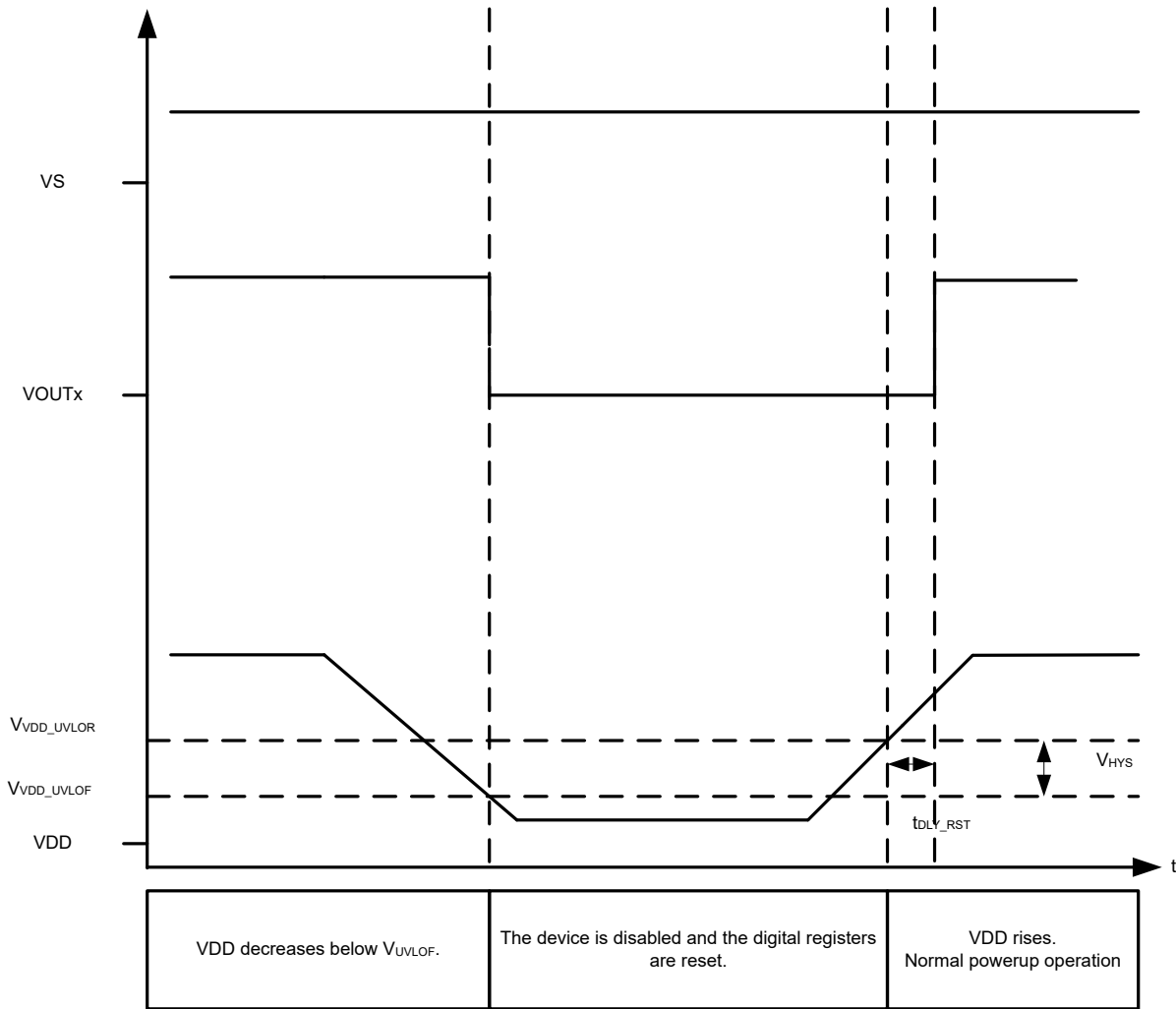
图 8-29. VDD UVLO
