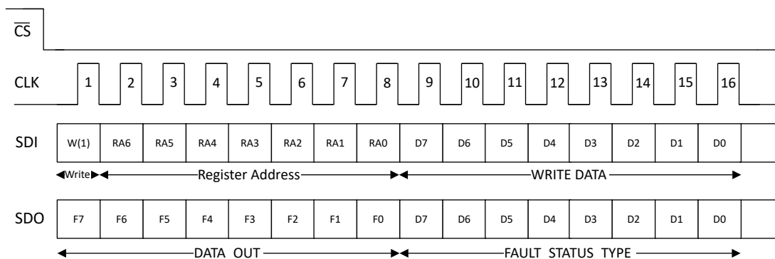
图 8-12. 16-bit Write, DSPI=1, D24BIT=0, CRC_EN=0
