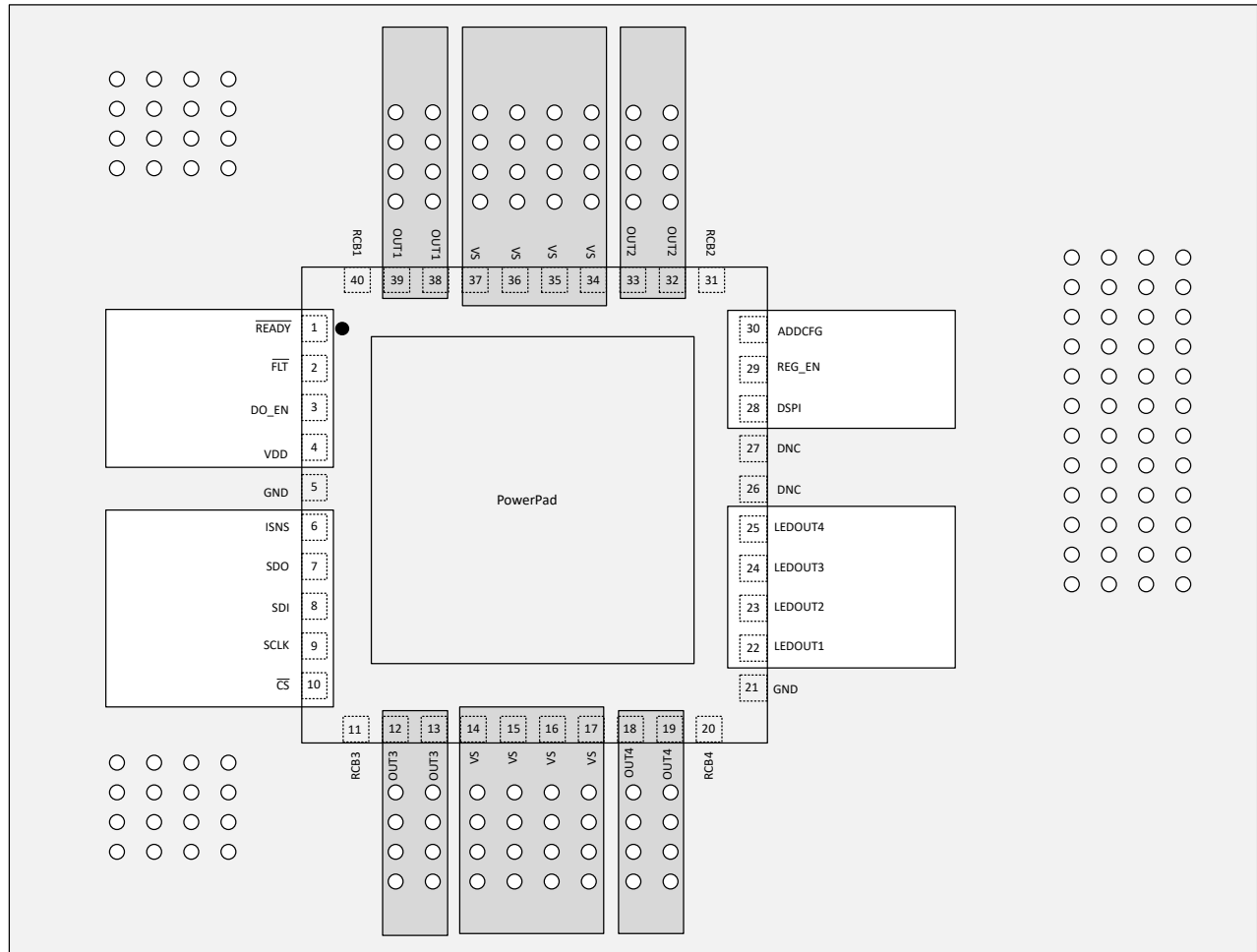
图 9-4. Layout Example
