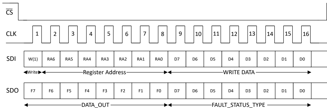
图 8-12. 16-bit Write, DSPI=1, D24BIT=0, CRC_EN=0
