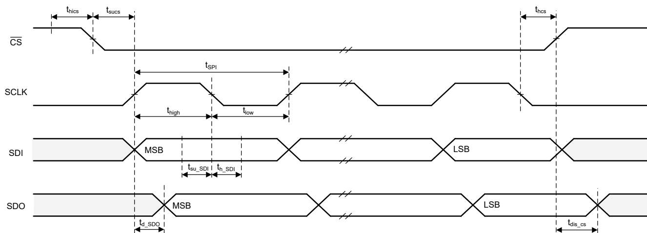
图 7-2. SPI Timing
