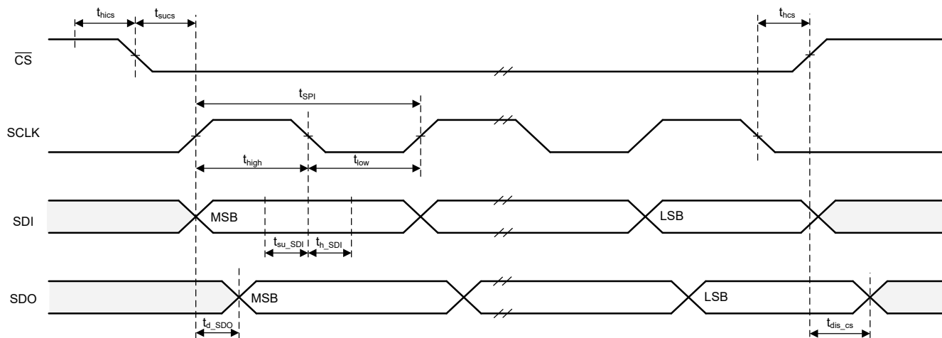
图 7-2. SPI Timing
