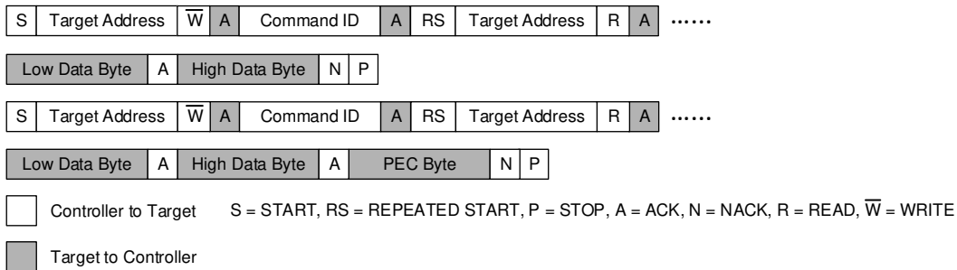
图 8-15. Read Word
