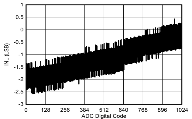
图 7-24. ADC INL
