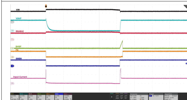
图 7-43. Power Down Using EN With Output Discharge
