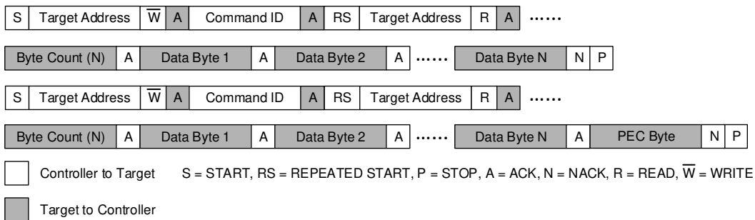
图 8-16. Block Read
