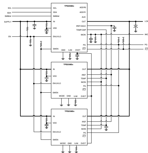
简化原理图
