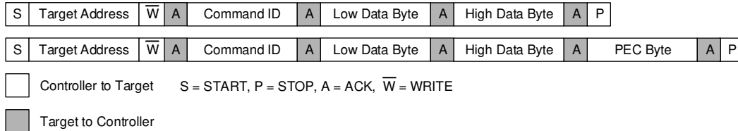
图 8-14. Write Word
