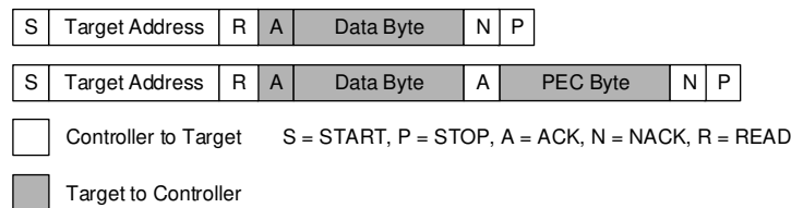
图 8-11. Receive Byte
