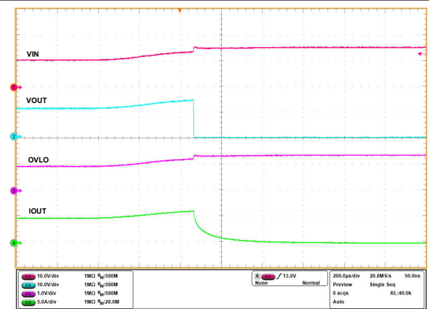
图 6-24. 过压保护
