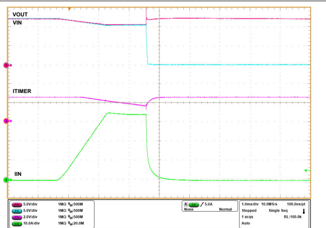
图 6-26. 稳态电流限制响应 (TPS259830L 型号)
