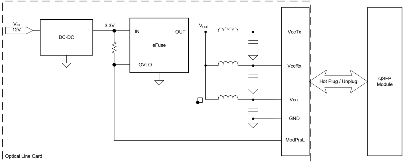
图 8-10. 典型光学线路卡的电源树方框图
