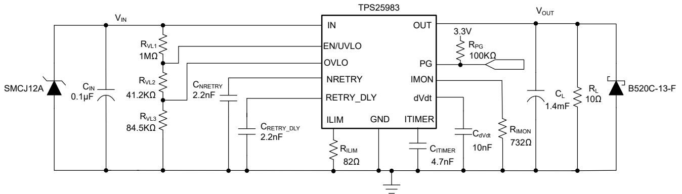
图 8-1. 典型应用原理图 - 保护服务器待机电源轨
