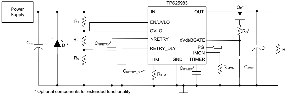
简化版原理图
