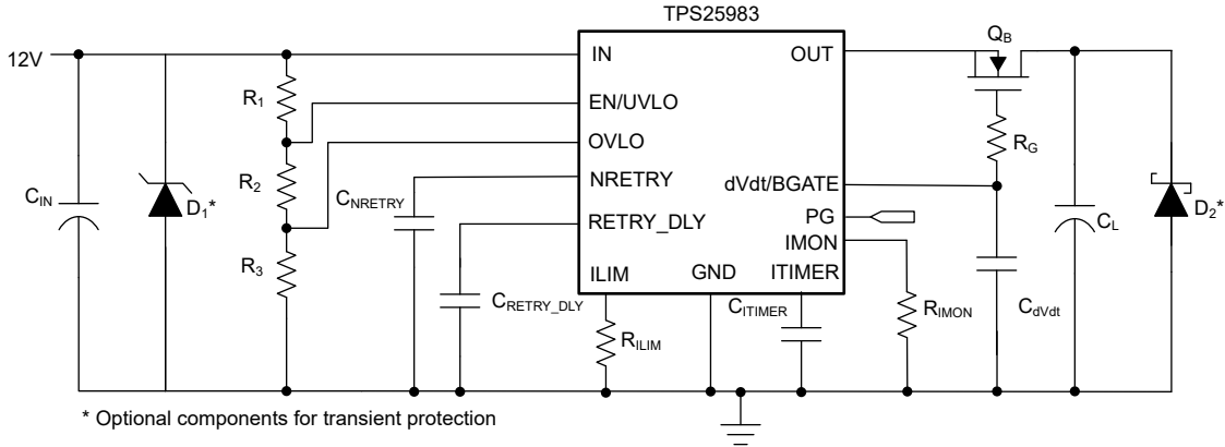
图 8-20. 采用可选保护元件的典型电路实施方案
