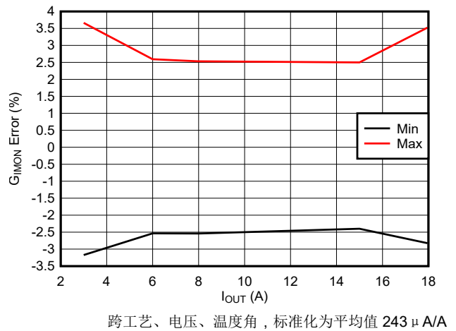
图 6-12. 输出电流监测器增益 ( G_{\text{IMON}} ) 精度
