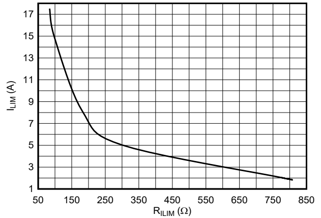
图 6-10. 输出电流限制 ( I_{\text{LIM}} ) 与 R_{\text{LIM}} 间的关系
