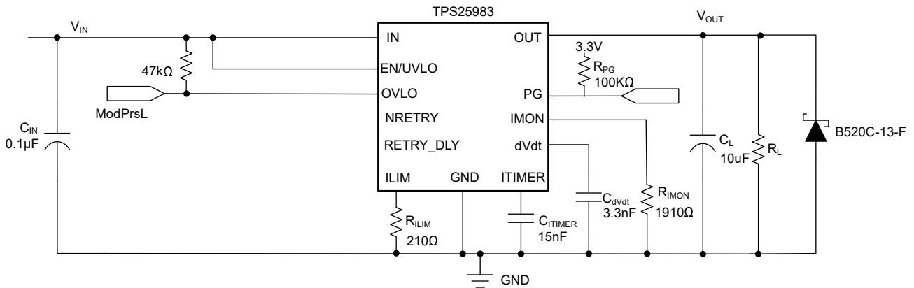
图 8-11. 在光学模块中配置用于 3.3V 电源轨路径保护的 TPS2598300
