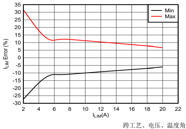
图 6-11. 输出电流限制 ( I_{\text{LIM}} ) 精度
