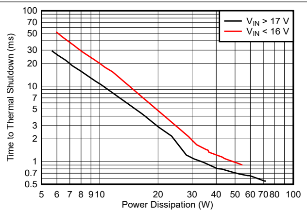
图 6-20. 热关断图 - 浪涌/过载
