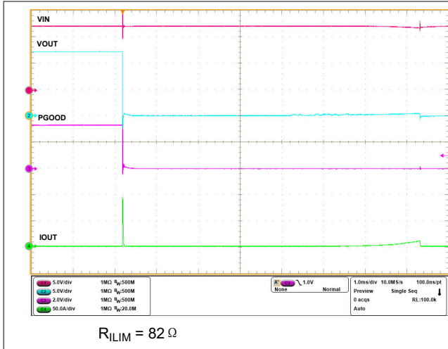
图 8-7. 导通时输出硬短路
