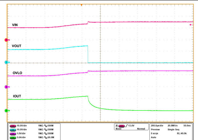
图 6-24. 过压保护
