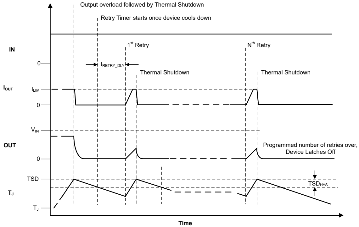
图 7-10. 故障后自动重试
