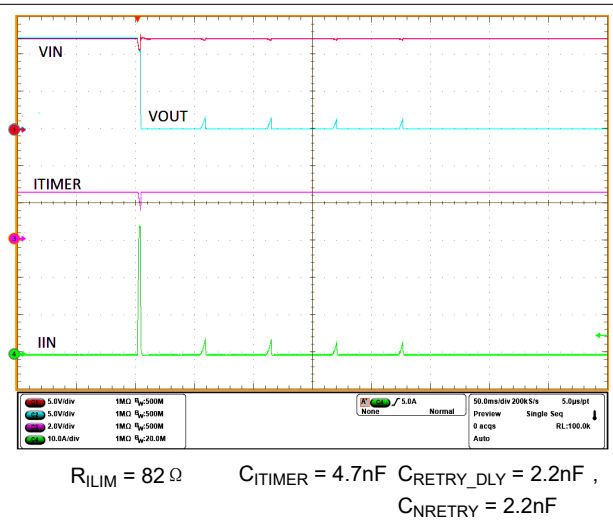
图 8-6. 断路器自动重试 4 次，重试延迟为 100ms
