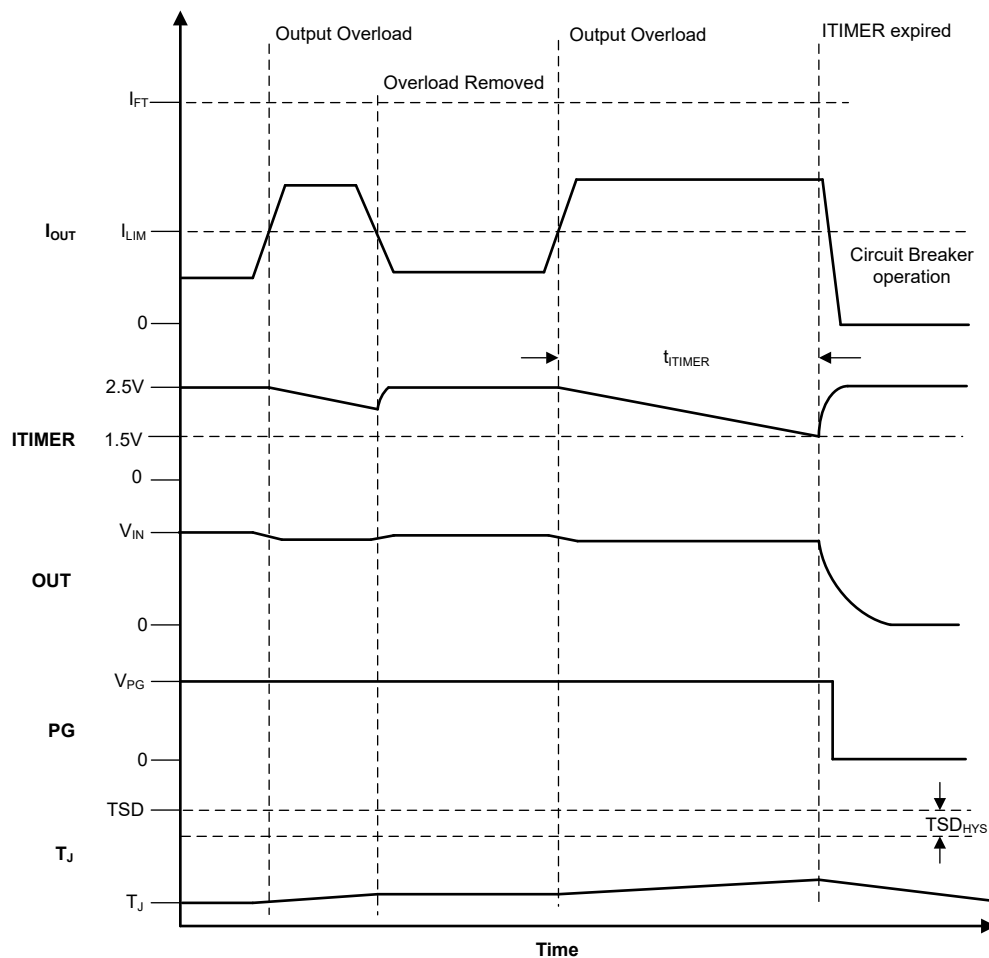
图 7-4. 断路器响应
