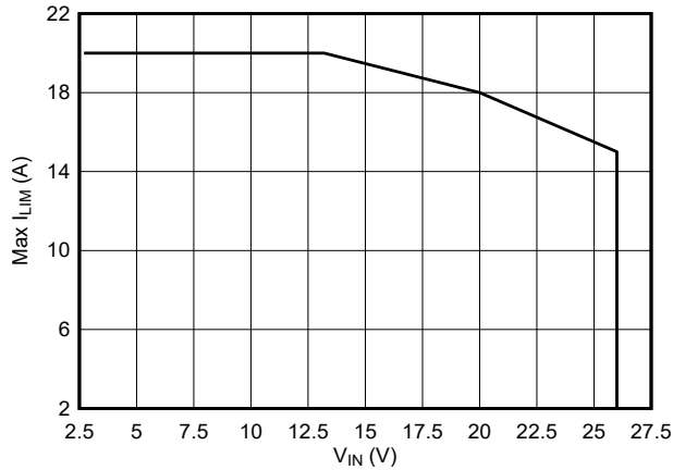
图 6-9. 安全运行的建议最大 I_{\text{LIM}} 设置与输入电压间的关系
