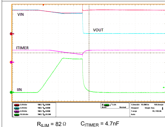
图 8-5. 具有 2ms 瞬态过流消隐间隔的断路器
