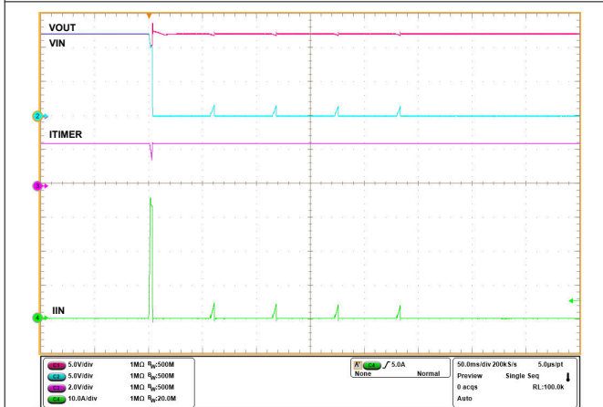
图 6-25. 瞬态过流消隐计时器响应
