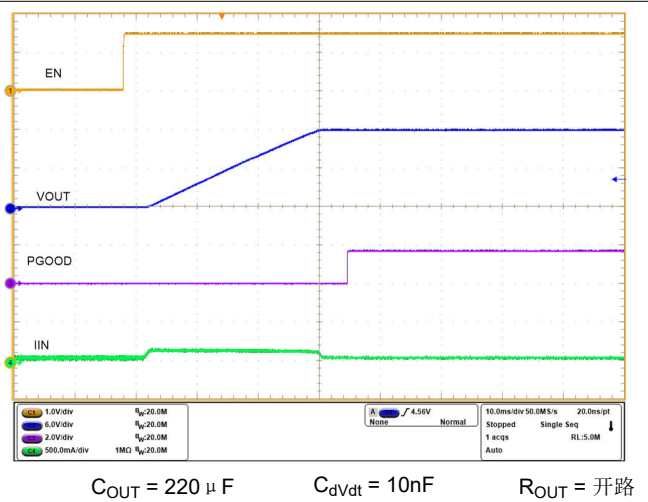
图 6-22. 通过 EN 启动 - dVdt 受限
