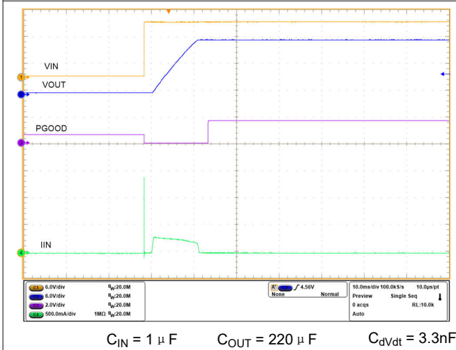
图 6-21. 热插拔
