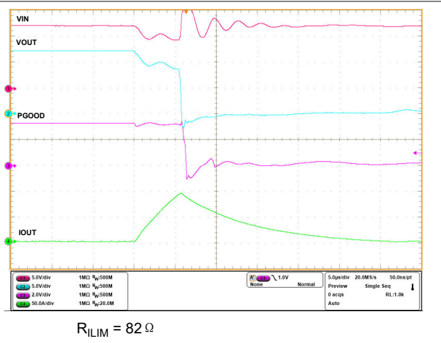
图 8-8. 导通时输出硬短路 (放大图)
