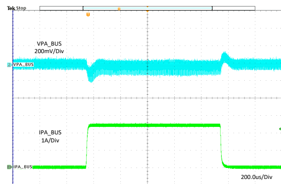
图 11-5. Load Regulation
