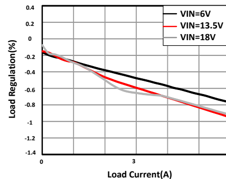
图 11-5. Load Regulation
