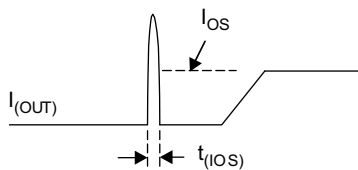
图 9-5. Output Short-Circuit Parameters
