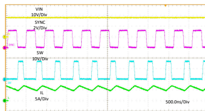
VIN = 18 V L = 0.68 uH I PA_BUS = 3 A I PB_BUS = 3 A
