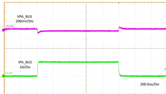
图 11-5. Load Regulation
