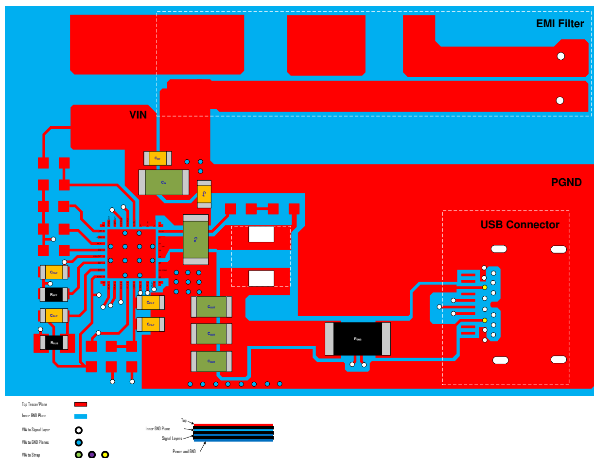
图 13-1. Layout
