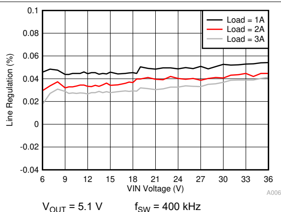
图 11-7. Line Regulation
