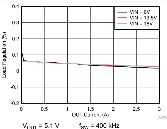
图 11-6. Load Regulation
