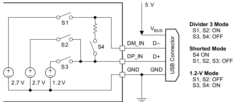
图 10-35. DCP Auto Mode
