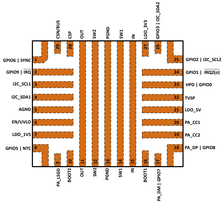
图 5-1. RQFN 封装 29 引脚 (VQFN) 顶视图
