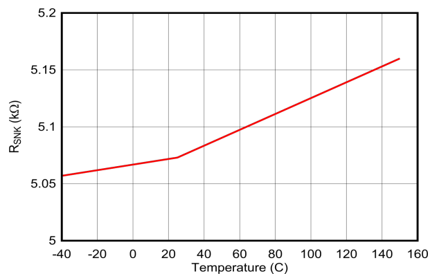
图 6-38. Type-C 电缆检测: R_{Snk} 与温度间的关系
