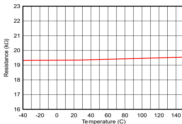
图 6-42. USB BC1.2: DM 至 AGND 20kΩ 电阻 R_{DM\_DWN\_20k}
