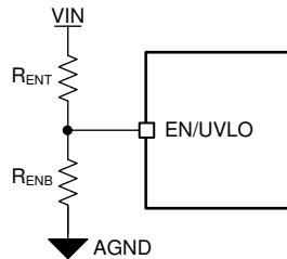
图 8-2. UVLO 阈值编程
