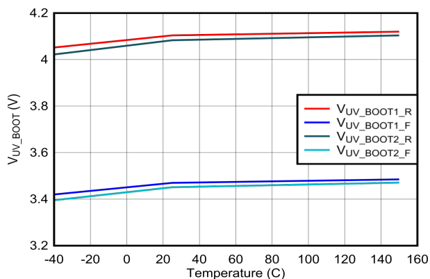
图 6-22. BOOTx UVLO 与温度间的关系
