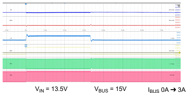
图 9-32. 负载瞬态 (降压/升压) : V_{BUS} = 15V
