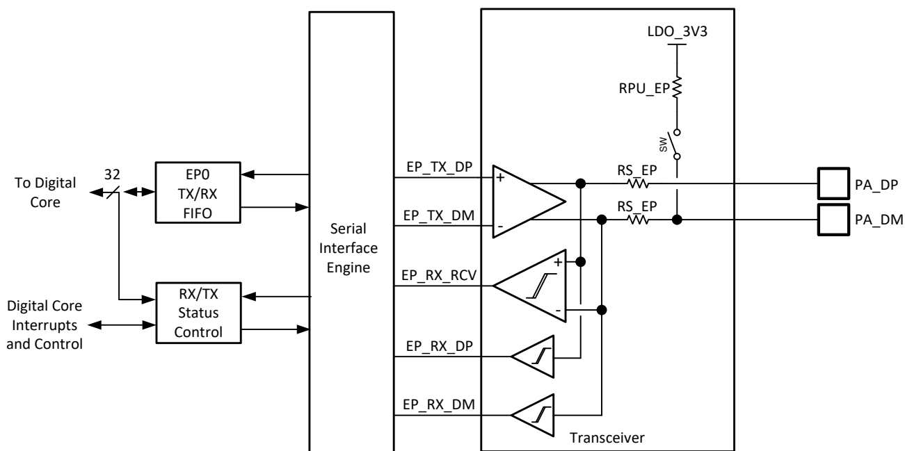
图 8-33. USB 端点 PHY
