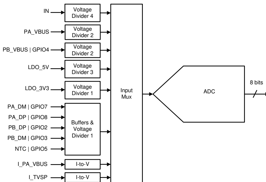
图 8-30. SAR ADC
