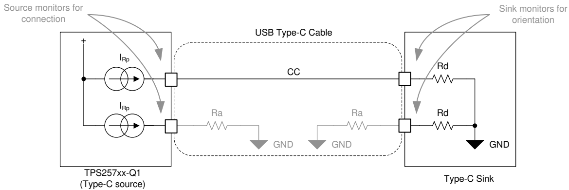
图 8-28. Type-C 电缆
