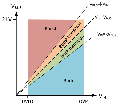
图 8-12. 工作区域
