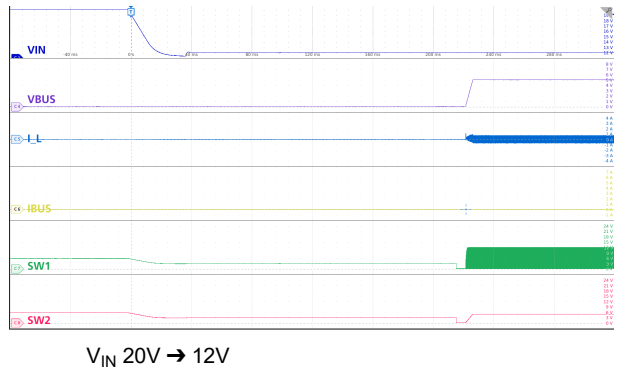
图 9-28. V_{IN(OVP)} 恢复
