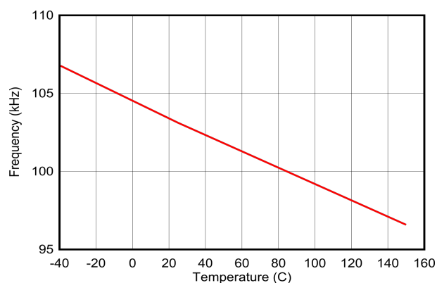
图 6-36. (M0) 100kHz 振荡器与温度间的关系
