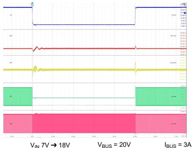
图 9-35. 线路瞬态： V_{BUS} = 20V
