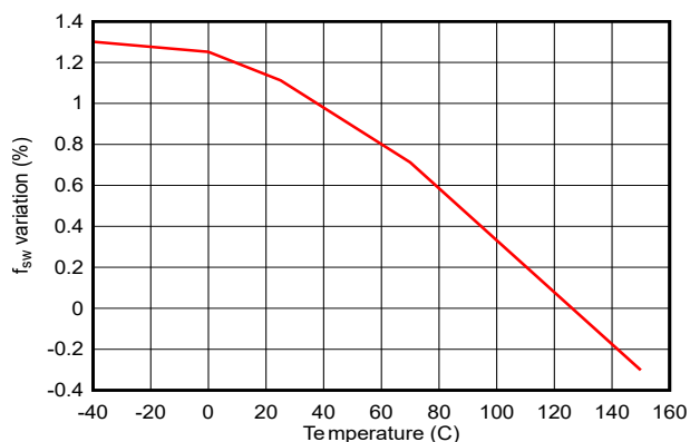
图 6-24. 降压/升压开关频率变化与温度间的关系 与标称值相比的百分比变化
