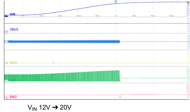
图 9-27. V_{IN(OVP)} 进入
