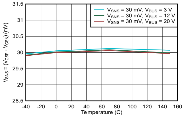
图 6-27. 电流环路调节电压与 V_{BUS} 和温度间的关系
