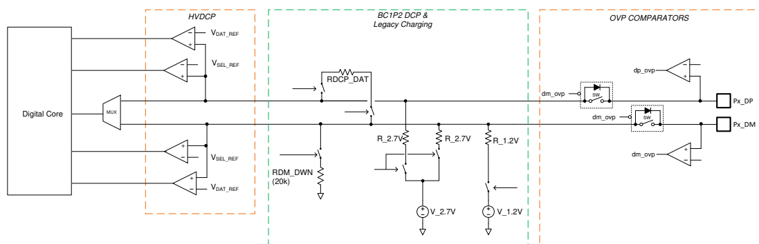
图 8-32. BC1P2 功能框图
