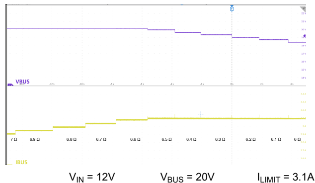
图 9-34. 电流限制：阶梯型阻性负载
