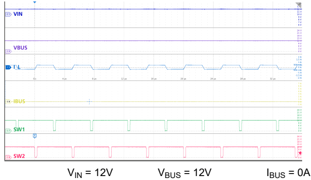
图 9-22. 降压/升压模式： V_{IN} = V_{BUS} ，空载
