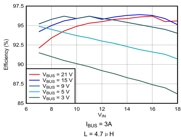
图 9-11. 效率与输入电压之间的关系
