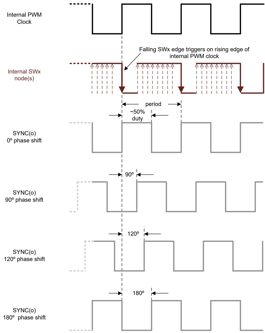
图 8-14. SYNC(o) 相移
