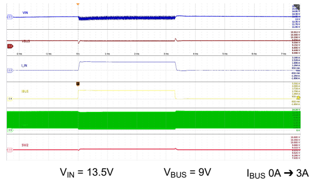
图 9-31. 负载瞬态 (降压) : V_{BUS} = 9V
