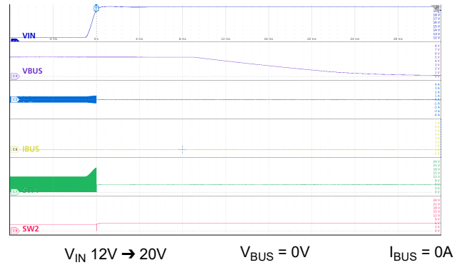
图 9-29. V_{IN(OVP)} 显示 V_{BUS} 放电
