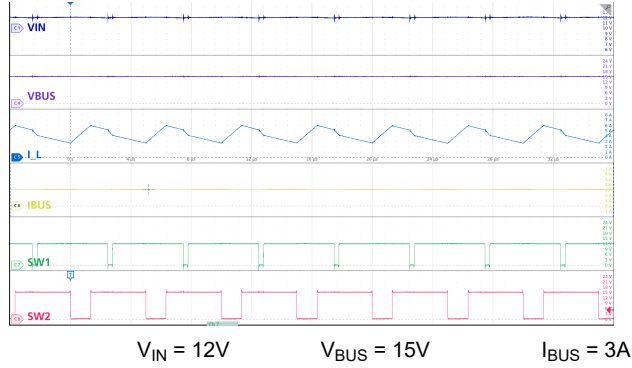
图 9-26. 降压/升压模式：标称 V_{IN} ，3A 负载
