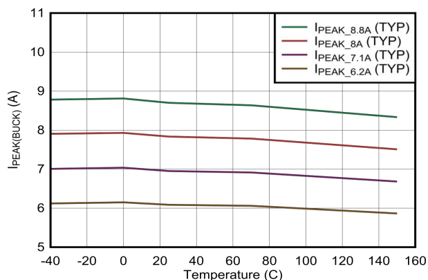
图 6-20. 降压峰值电流限制与温度间的关系 (下限设置)
