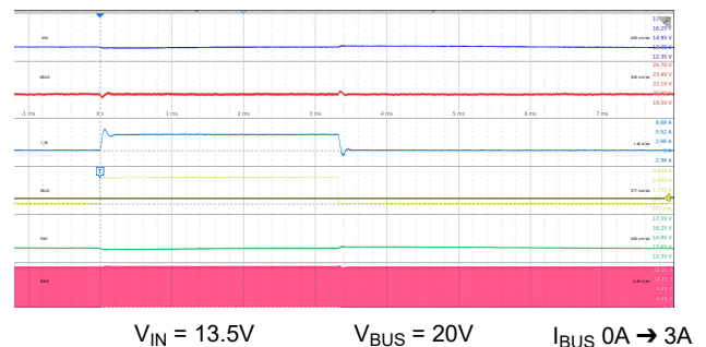
图 9-33. 负载瞬态 (升压) : V_{BUS} = 20V
