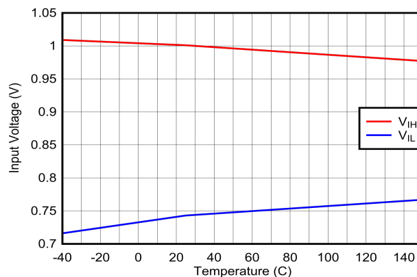
图 6-48. GPIO : 输入电压阈值与温度间的关系
