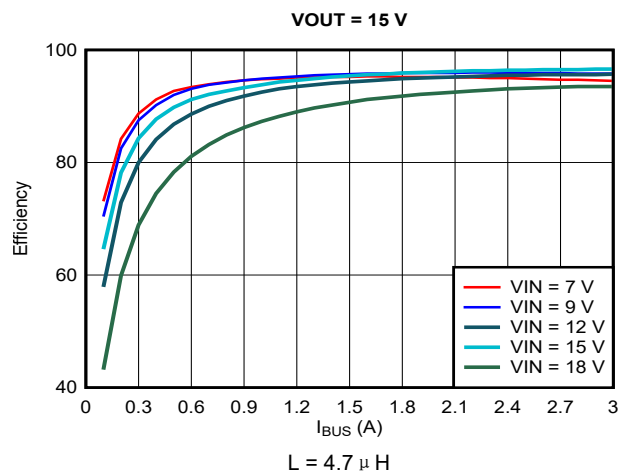
图 9-9. 效率与输出电流 ( I_{OUT} ) 间的关系, V_{OUT} = 15V
