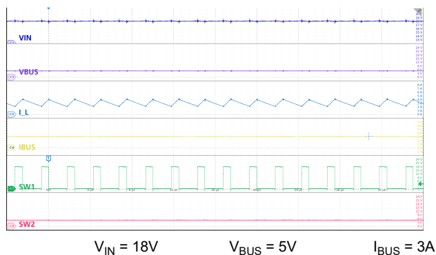
图 9-17. 降压模式：高 V_{IN} ，3A 负载
