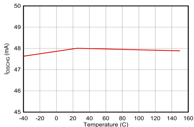
图 6-34. V_{BUS} 放电电流与温度间的关系
