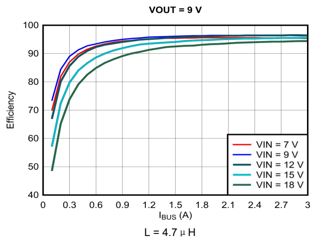
图 9-7. 效率与输出电流 ( I_{OUT} ) 间的关系, V_{OUT} = 9V
