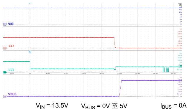
图 9-12. Type-C 连接
