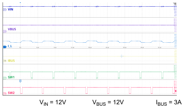
图 9-24. 降压/升压模式： V_{IN} = V_{BUS} ，3A 负载
