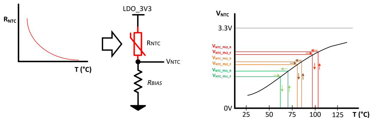
图 8-43. NTC 响应曲线
