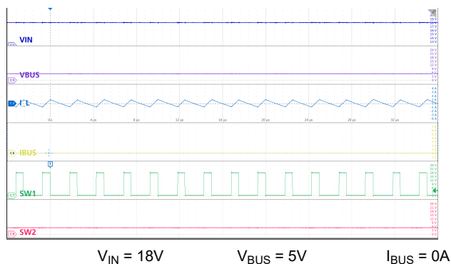
图 9-15. 降压模式：高 V_{IN} ，空载
