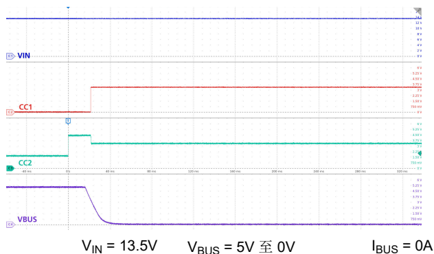
图 9-13. Type-C 断开
