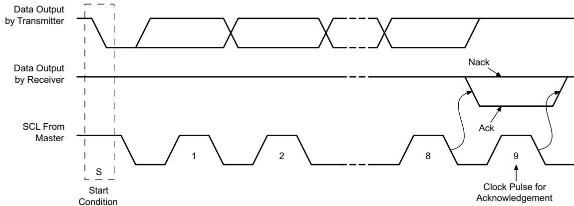
图 8-37. I 2 C 确认
