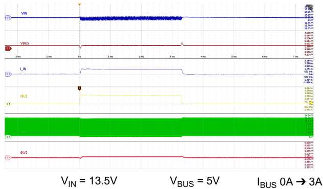
图 9-30. 负载瞬态 (降压) : V_{BUS} = 5V
