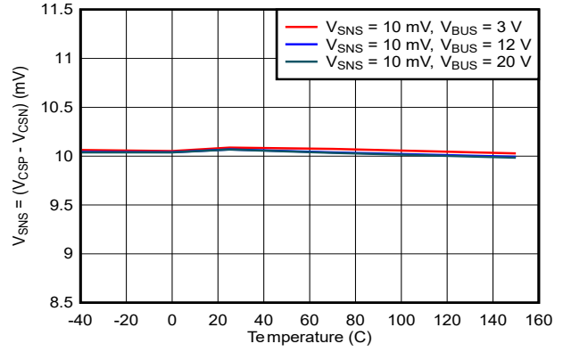
图 6-26. 电流环路调节电压与 V_{BUS} 和温度间的关系
