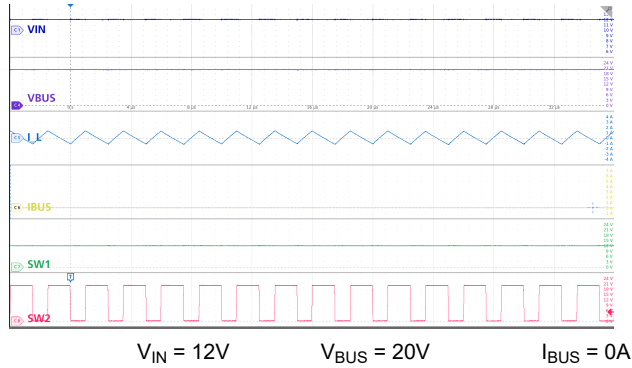
图 9-18. 升压模式：标称 V_{IN} ，空载
