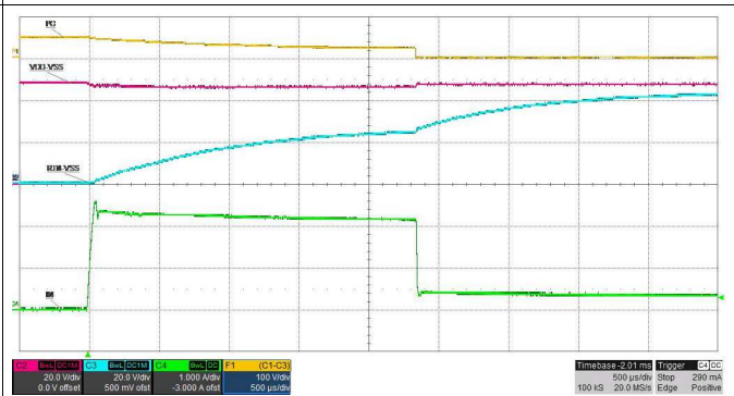
Figure 27. 过流响应
