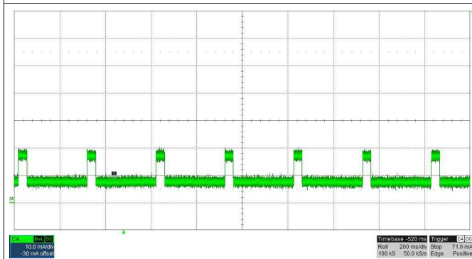
Figure 26. 自动 MPS
