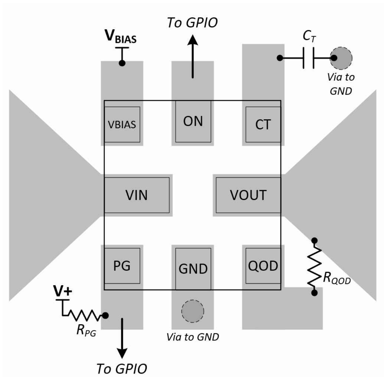
图 12-1. TPS22992x Layout Example
