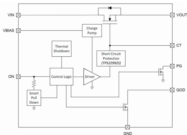
TPS22992x 方框图
